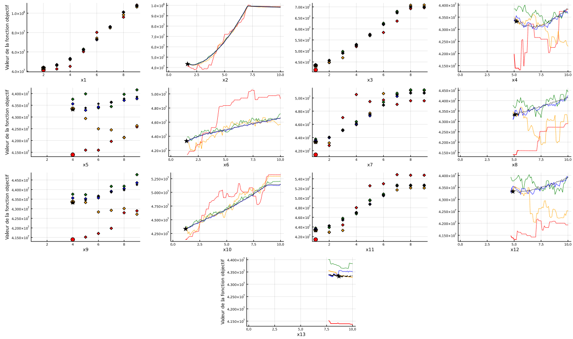
Figure 1: Graphiques de comportement de Micro-PRIAD pour l'instance 3 avec 13 entrées
