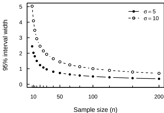
(d) Precision vs. noise
