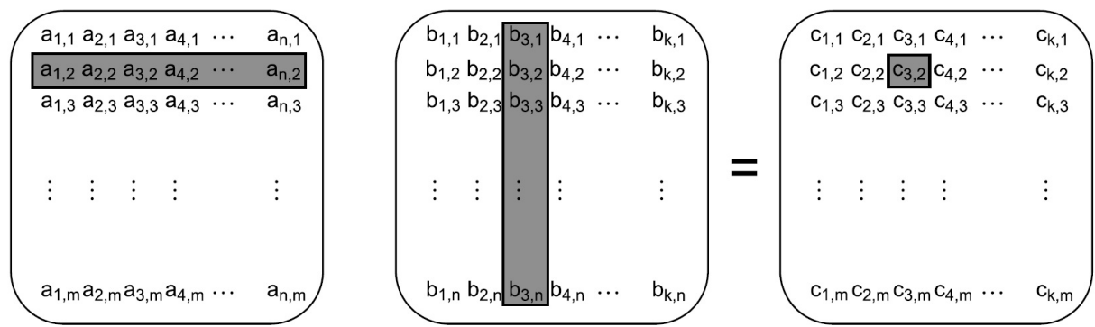
图8.3 矩阵相乘
