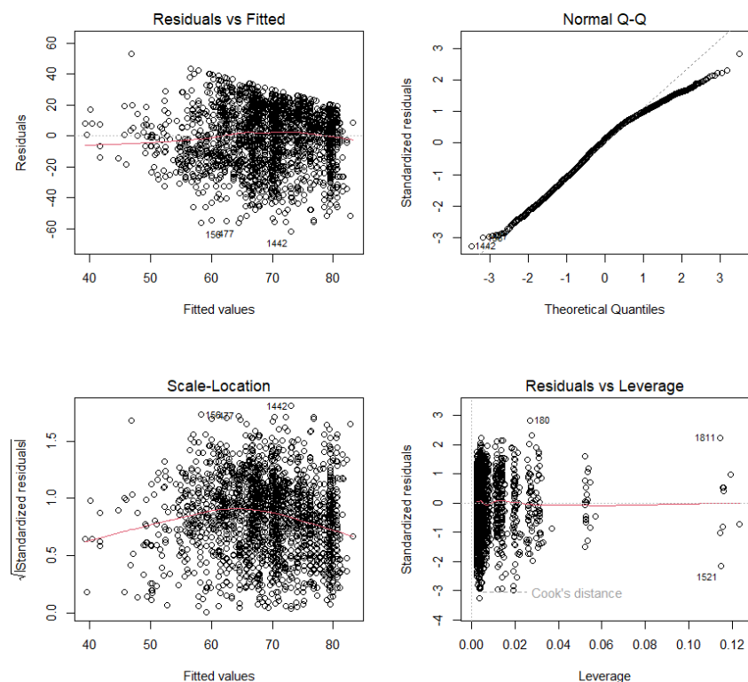
Figuur 1: Diagnostische plots voor het regressiemodel
