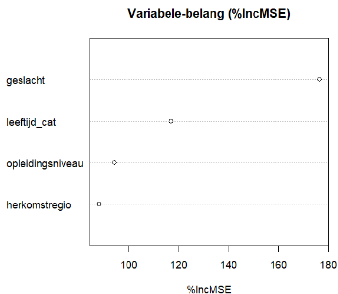
Figuur 4: Variabele-belang van het random woud
