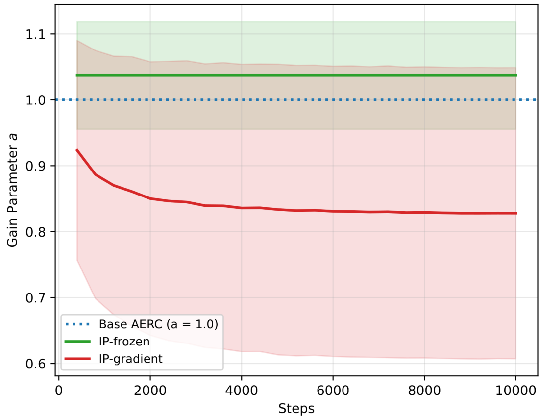
IP Gain a Parameter Evolution
