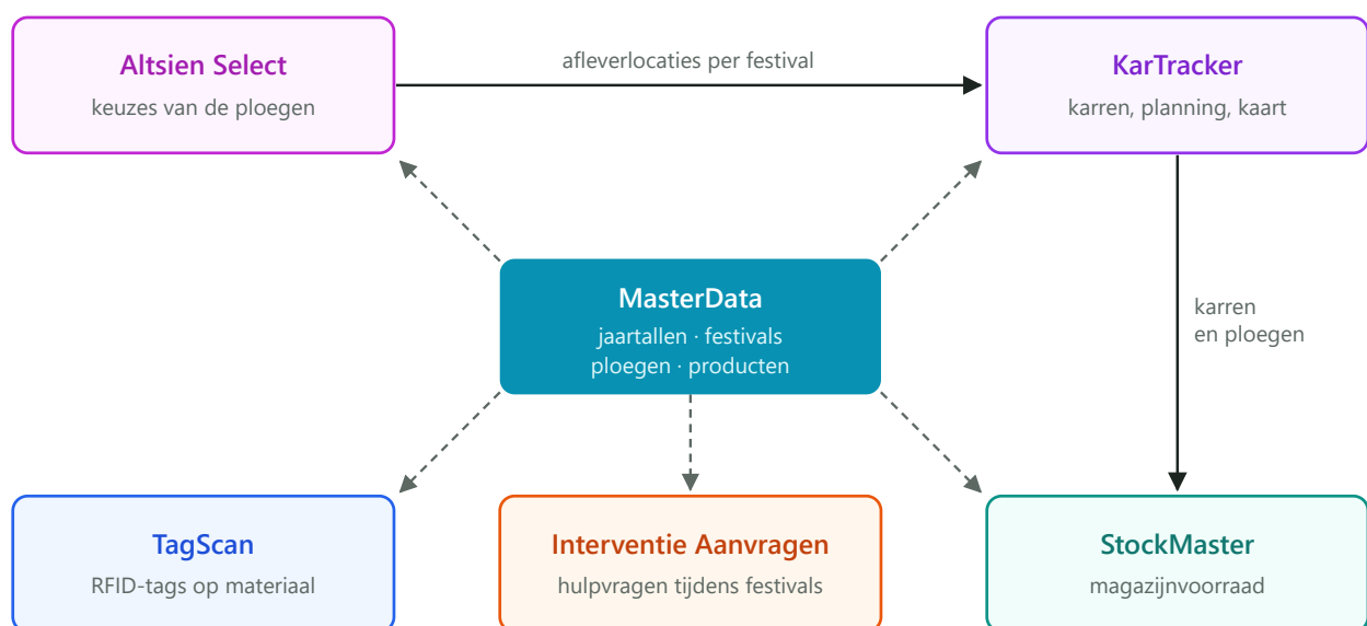
Figuur 1.1 – MasterData levert de basisgegevens aan alle modules (stippelijnen); daarnaast geven sommige modules gegevens aan elkaar door (volle pijlen).
