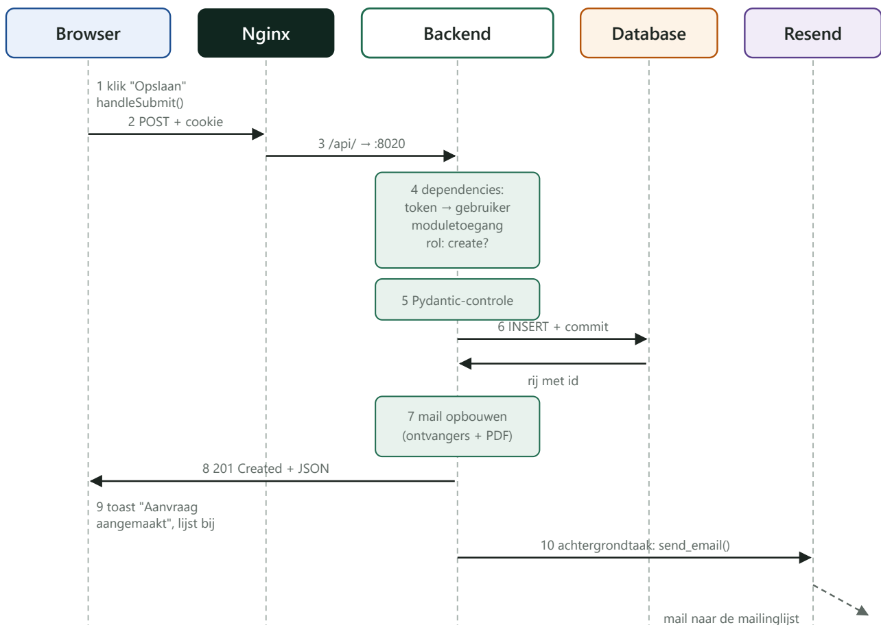
Figuur 13.1 – Het pad van "nieuwe interventie-aanvraag opslaan" door het systeem. De mail vertrekt pas nadat de gebruiker zijn antwoord kreeg.
