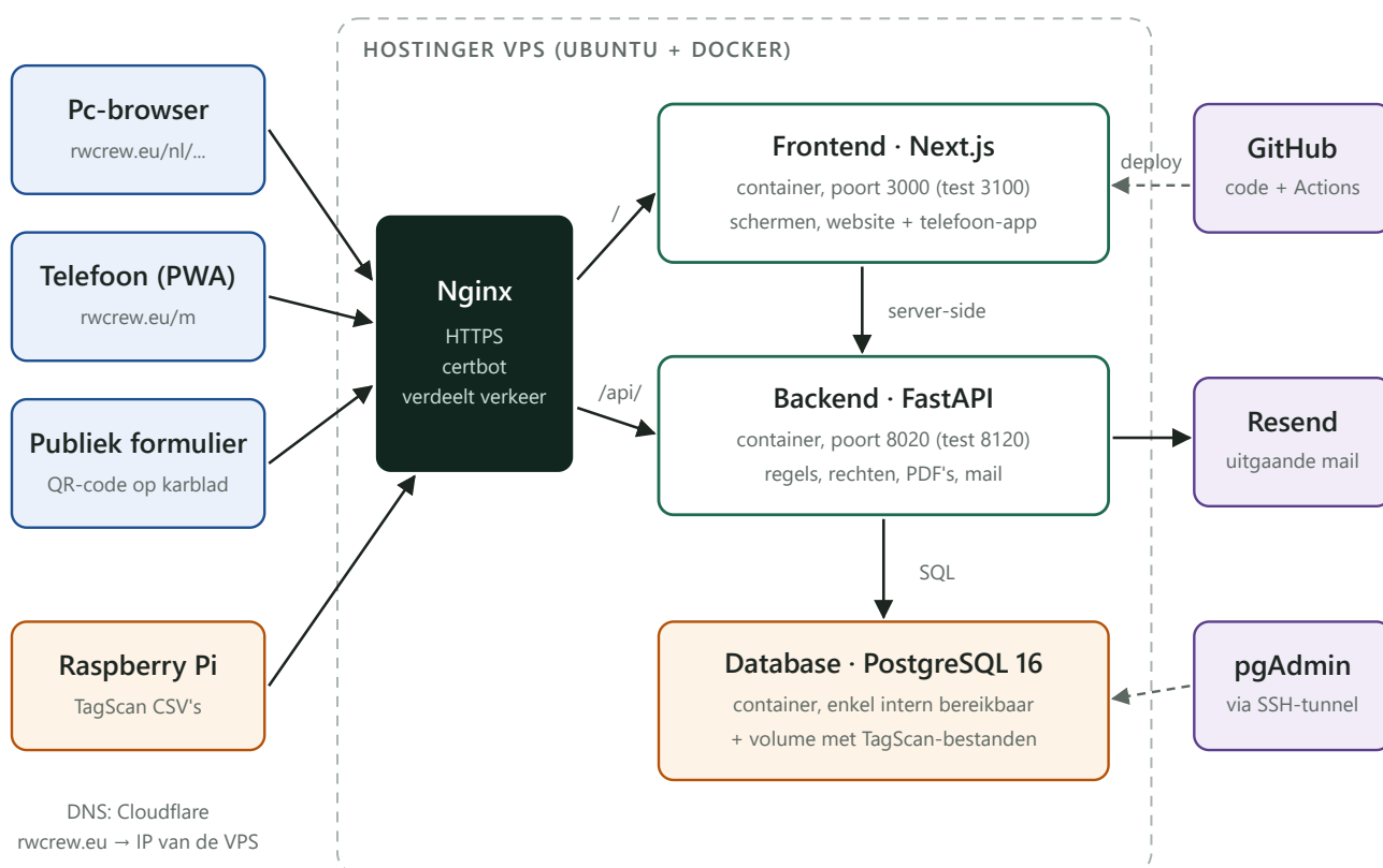
Figuur 4.1 – Overzicht van alle onderdelen van RWCrew en hun verbindingen (productie; test is een tweede, identieke set containers op dezelfde server).
