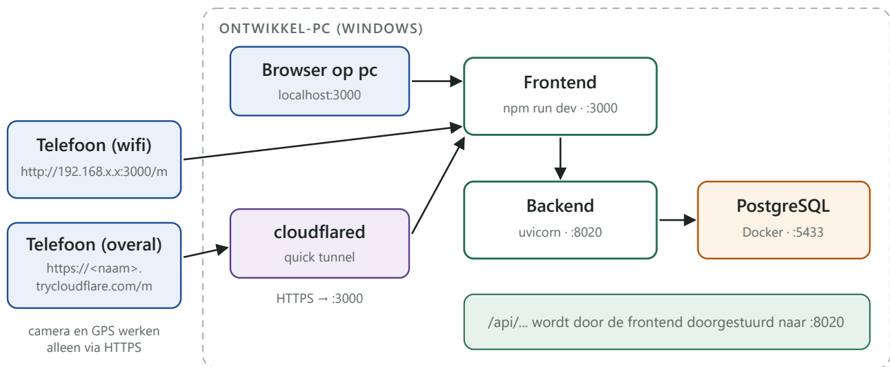
Figuur 5.1 – De lokale opstelling: database in Docker, backend en frontend rechtstreeks, optioneel een tunnel voor een telefoon via HTTPS.
