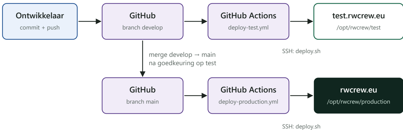
Figuur 6.1 – De weg van een wijziging: eerst naar test via develop , na controle naar productie via main .
