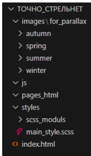
Рисунок 2.1 – Файловая структура
