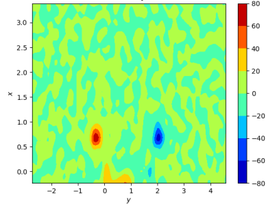
vorticity
