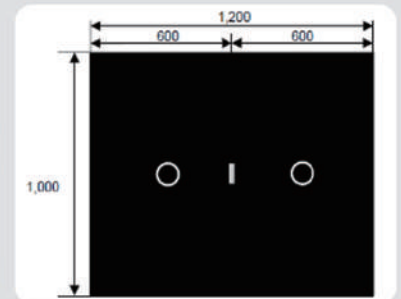
화스너 시공
