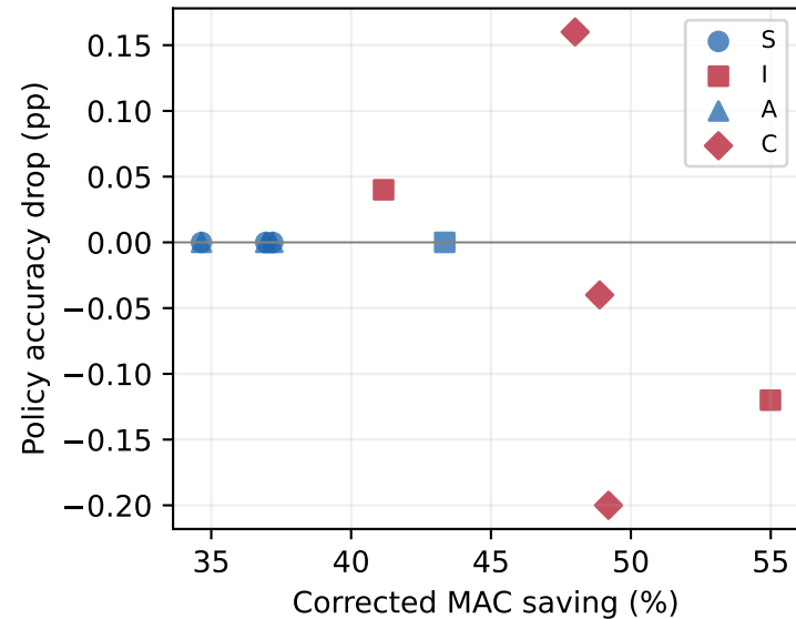
cifar10
