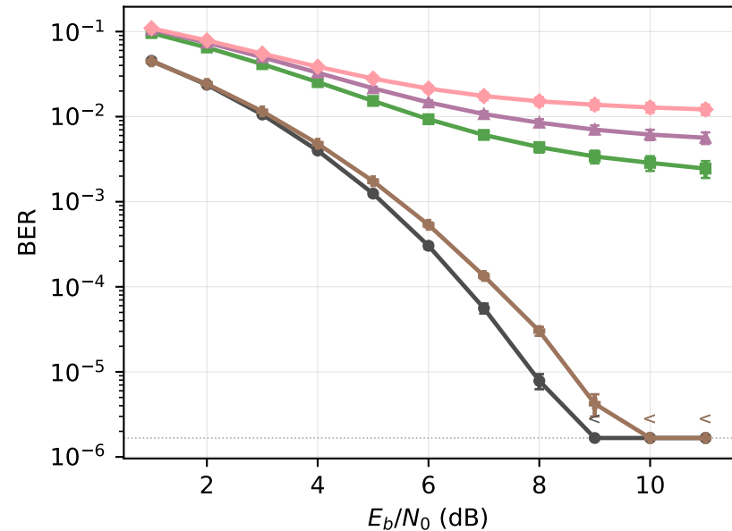
SSPA BER
