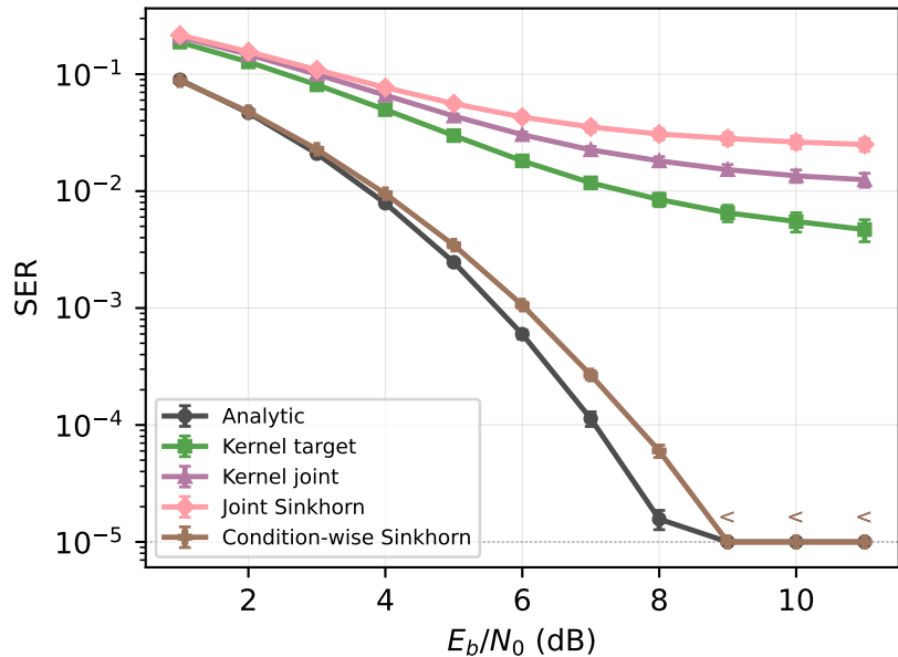
SSPA SER
