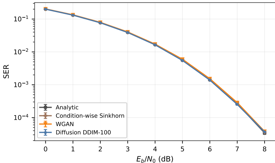
AWGN SER
