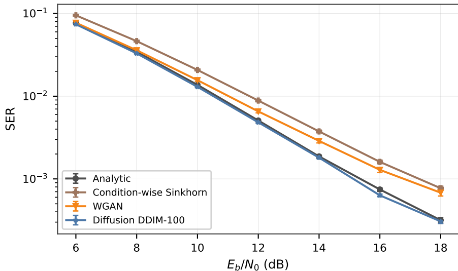
Rayleigh SER
