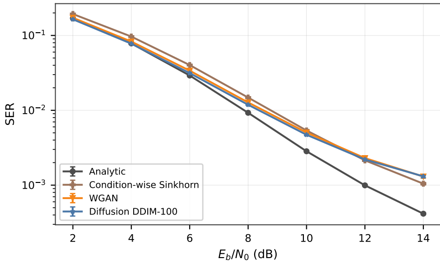
TDL SER
