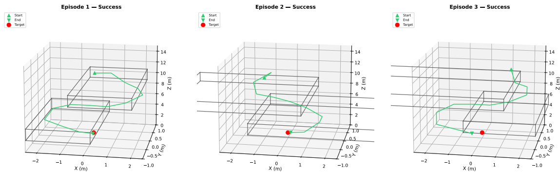
Abbildung 5.4.: Exemplarische 3D-Trajektorien dreier erfolgreicher Episoden in der Korridorumgebung. Die grauen Quader zeigen die achsenparallelen Begrenzungsboxen (AABB) der Hindernisse. Grünes Dreieck: Startposition bei z \approx 12 m, roter Punkt: Landeziel bei (0, 0, 1) m.
