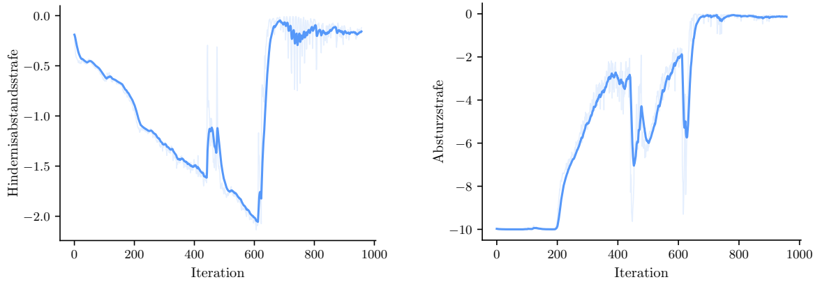
Abbildung A2.: Hindernisabstandsstrafe (links) und Absturzstrafe (rechts). Beide Strafkomponten fallen mit zunehmender Kollisionsvermeidung. Geglättet mit EMA \alpha = 0,9 .
