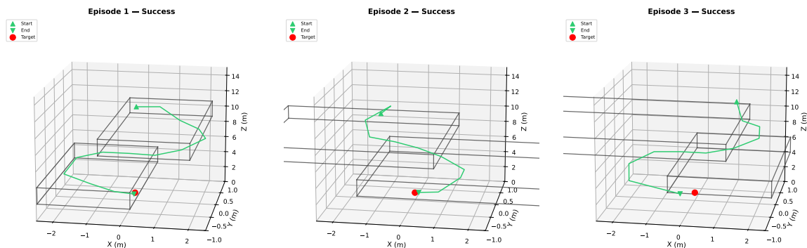
Abbildung 5.3.: Exemplarische 3D-Trajektorien dreier erfolgreicher Episoden. Graue Quader: AABB der Hindernisse. Grünes Dreieck: Startposition, roter Punkt: Landeziel.
