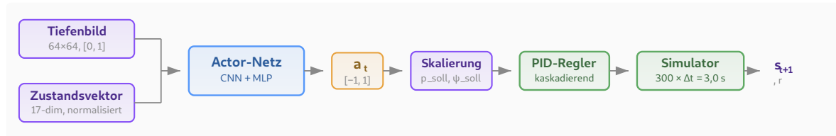
Abbildung 4.1.: Verarbeitungspipeline: Tiefenbild und Zustandsvektor werden dem Actor-Netz (CNN + MLP) übergeben, das eine Aktion sampelt. Nach Skalierung steuert ein kaskadierender PID-Regler die Drohne über 300 Simulationsschritte.
