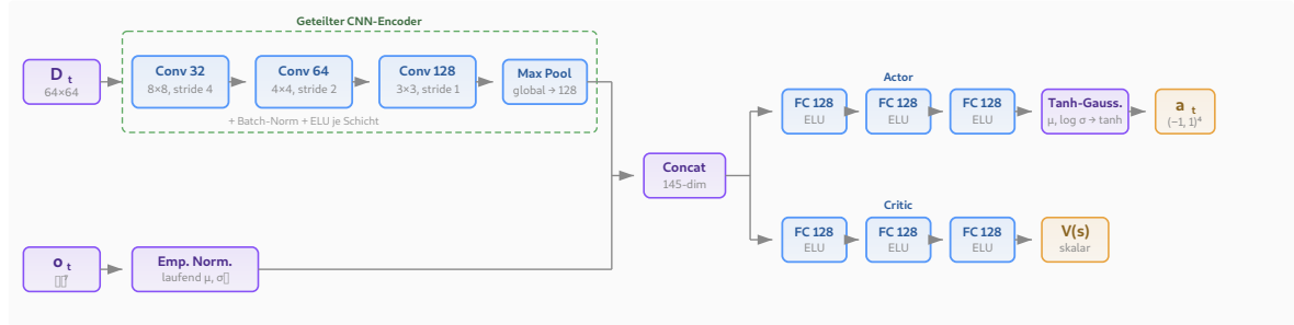
Abbildung 4.2.: Netzwerkarchitektur: Geteilter CNN-Encoder (drei Faltungsschichten mit Batch-Normalisierung, ELU und Global Max Pooling) erzeugt einen 128-dimensionalen Merkmalsvektor, der mit dem normalisierten Zustandsvektor konkateniert und an die getrennten MLP-Köpfe weitergegeben wird.
