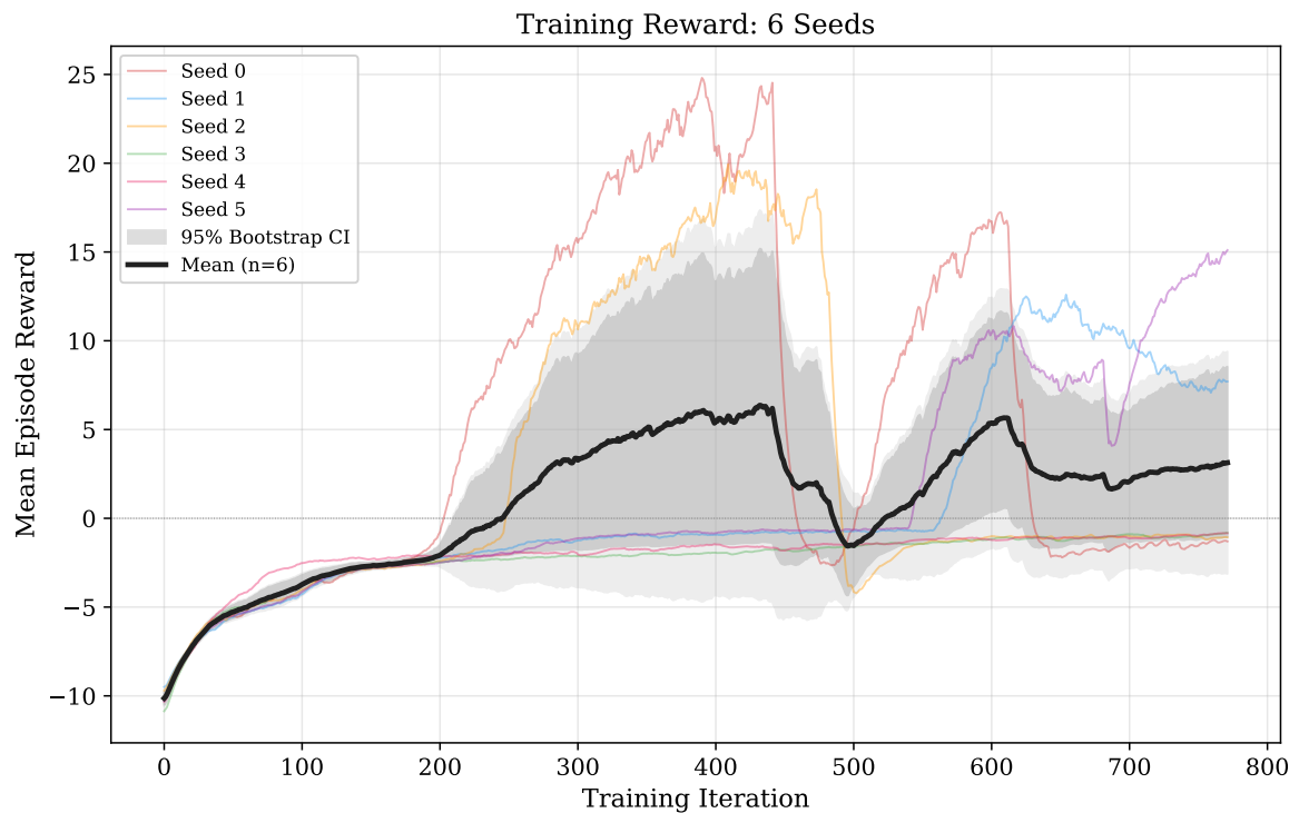
Abbildung 5.1.: Kumulative Belohnung über 6 Seeds mit identischen Hyperparametern. Schattierte Fläche: 95 %-Bootstrap-Konfidenzintervall des Mittelwerts (10 000 Resamples). EMA \alpha = 0,9 .
