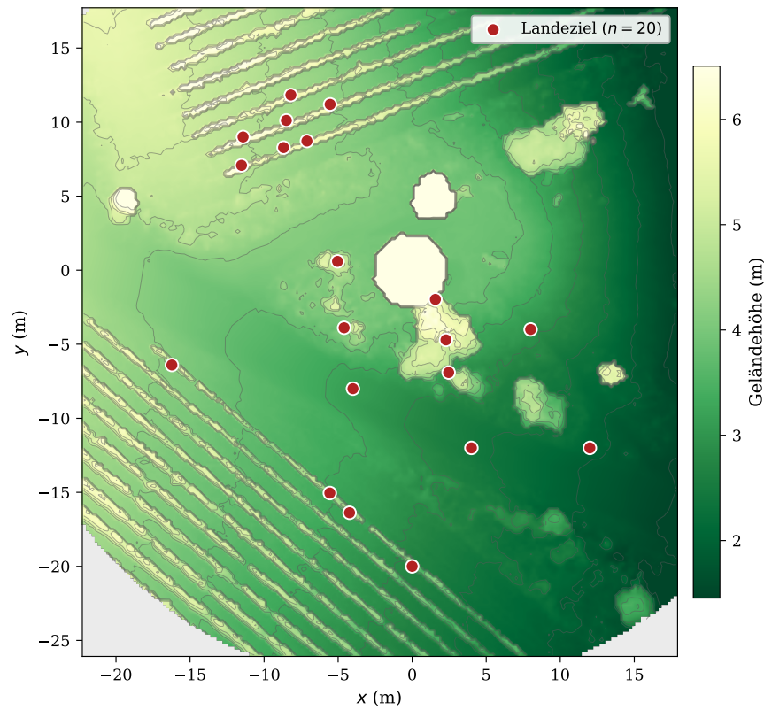
Abbildung 4.4.: Draufsicht auf das Höhenraster der Weinbergumgebung mit den 20 vordefinierten Zielpositionen. Die diagonalen Strukturen entsprechen den Rebenreihen.
