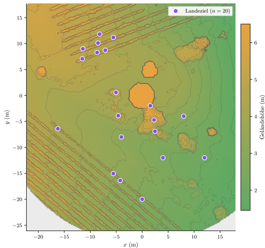
Abbildung 4.7.: Draufsicht auf das Höhenraster der Weinbergumgebung mit den 20 vordefinierten Zielpositionen. Die diagonalen Strukturen entsprechen den Reihen.
