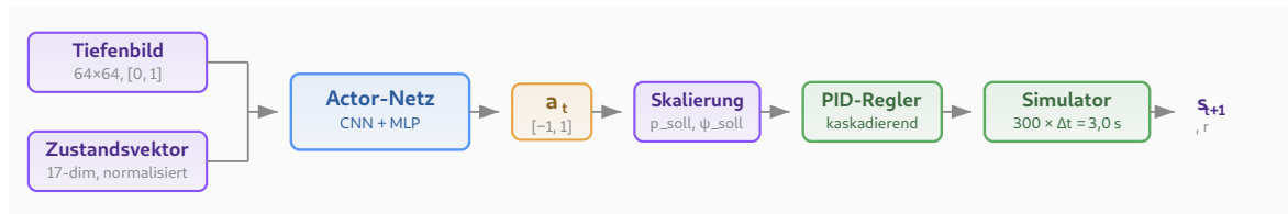
Abbildung 4.3.: Verarbeitungspipeline: Tiefenbild und Zustandsvektor werden dem Actor-Netz (CNN + MLP) übergeben, das eine Aktion sampelt. Nach Skalierung steuert ein kaskadierender PID-Regler die Drohne über 300 Simulationsschritte.
