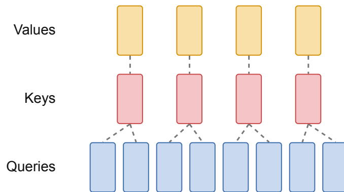
Grouped-Query Attention
