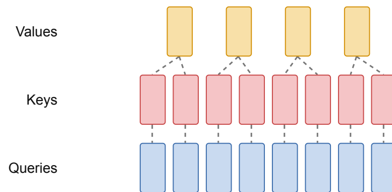
Grouped-Value Attention
