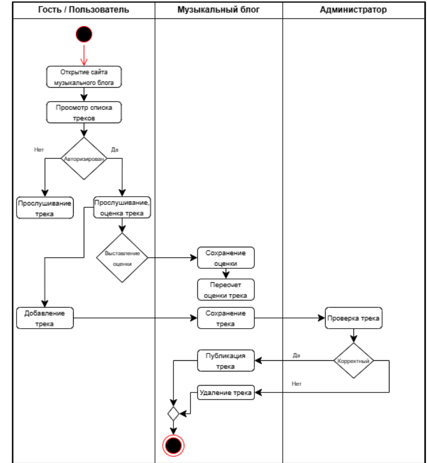
Диаграмма деятельности
