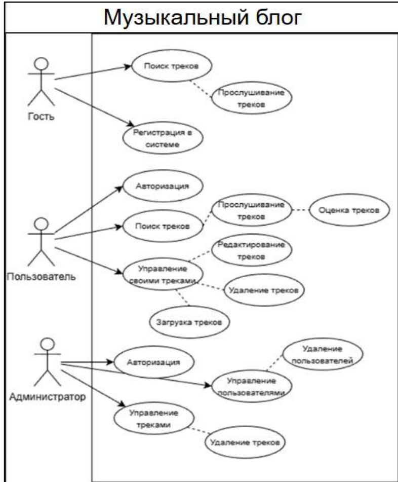
Диаграмма вариантов использования
