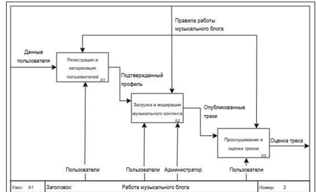
Диаграмма декомпозиций A1
