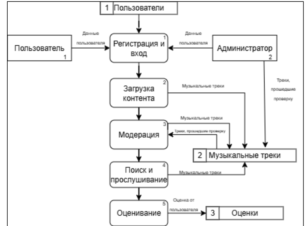
Диаграмма потоков данных
