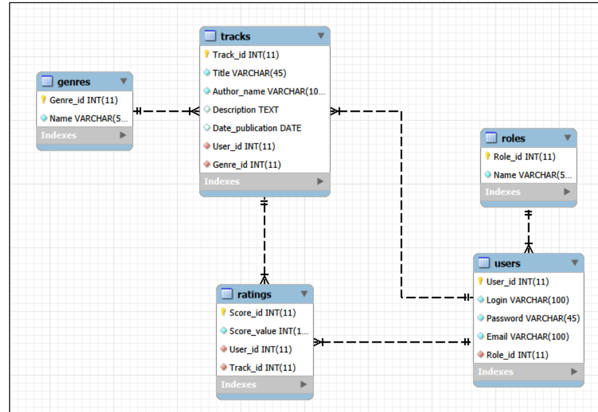
ER-Модель
