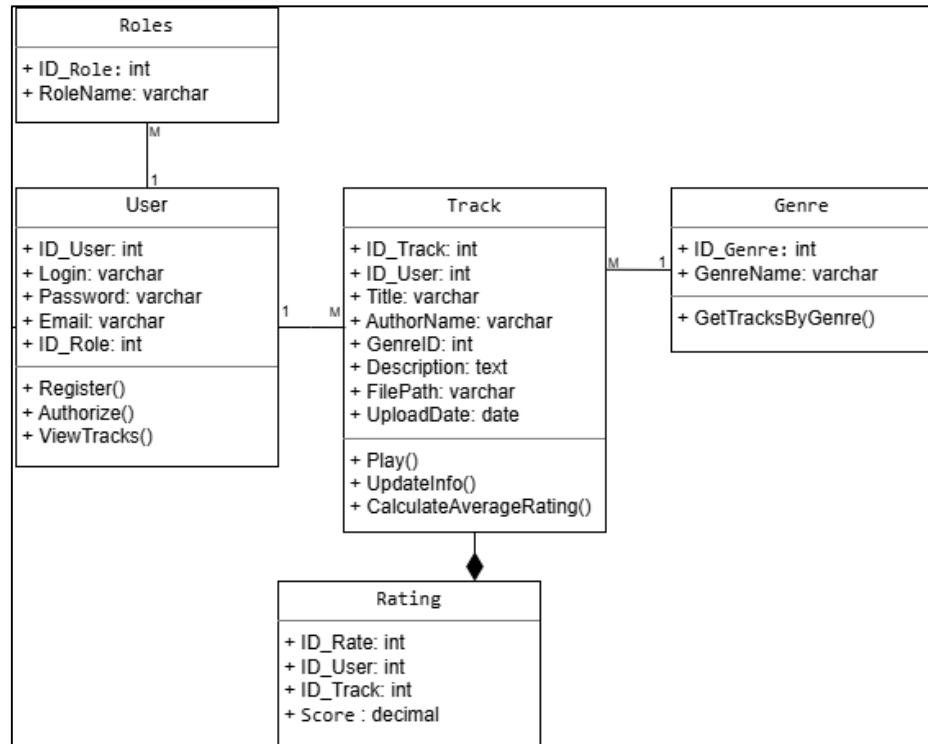
Диаграмма классов
