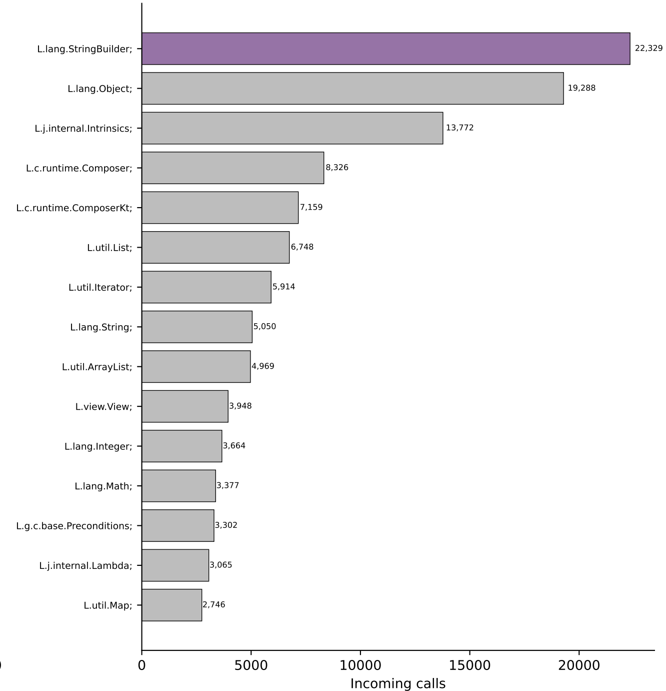
Top 15 Callees
