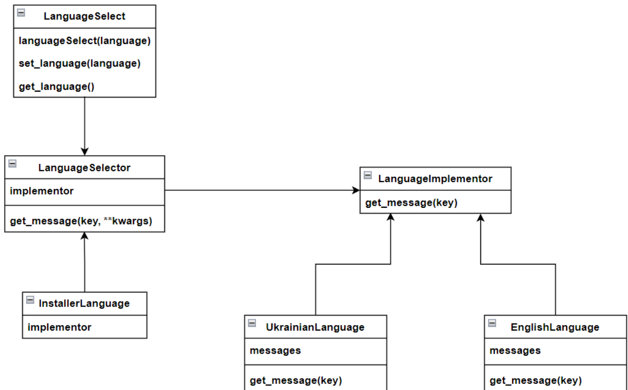
Рис. 3 – Діаграма класів для шаблону bridge
