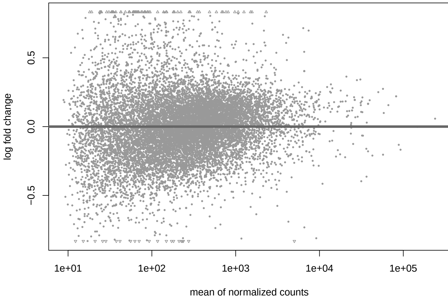
MA Plot: T3 vs T1
