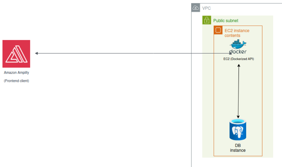
Figura 31 – Diagrama inicial da infraestrutura cloud do projeto WeConecta
