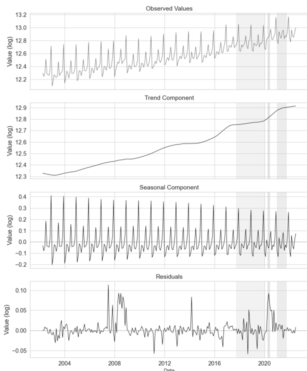
図 2: STL分解による時系列成分の分離
