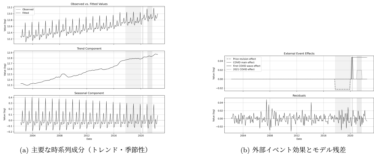
図 2: 提案モデルによる時系列成分の分解
