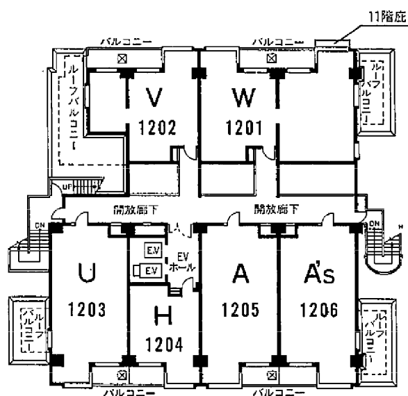
12階平面図
