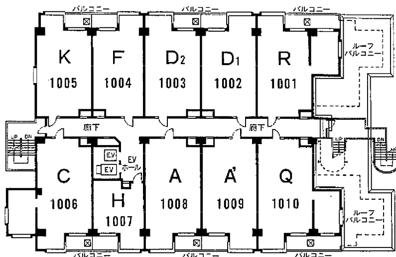
10階平面図
