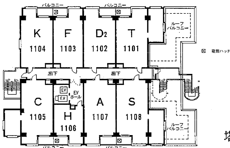
11階平面図
