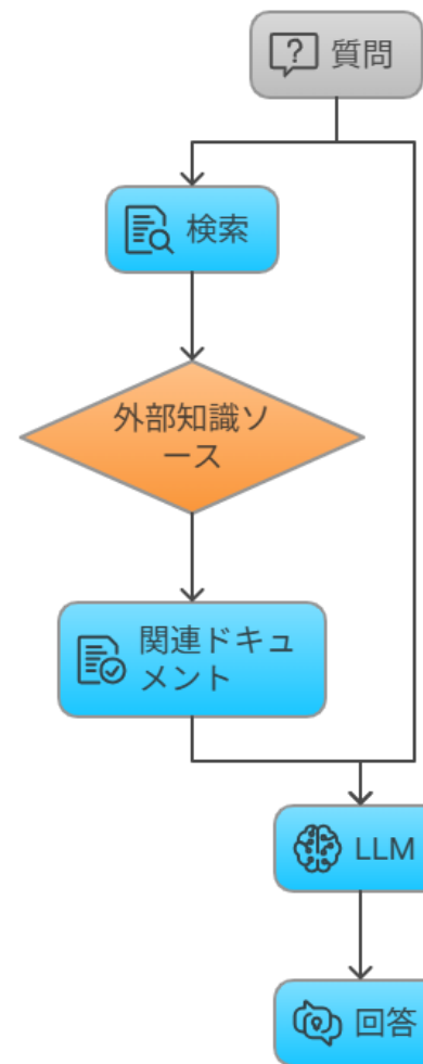
RAGの基本的な流れ
