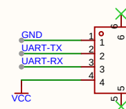
预留串口接口（复用为Modbus RTU 接口）
