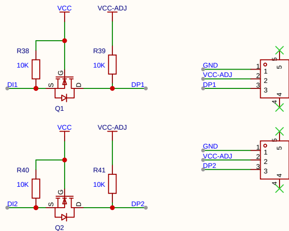
红外管拓展接口
