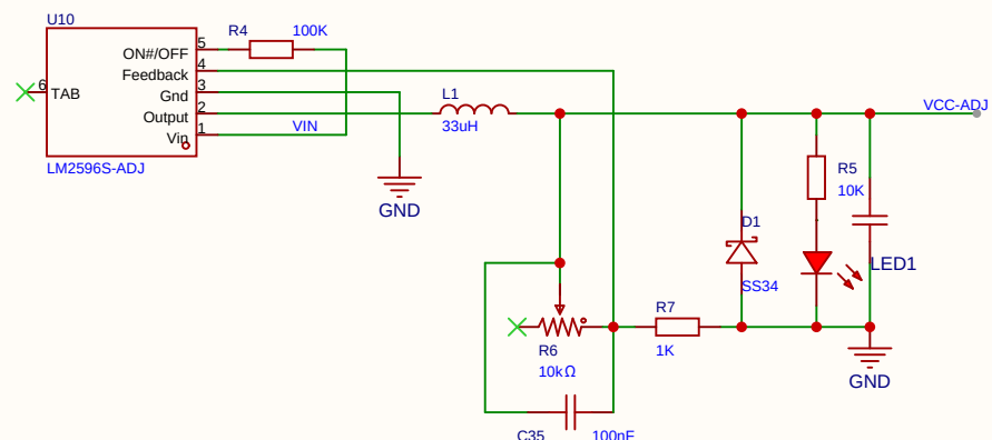
可调电源&输入电压检测
