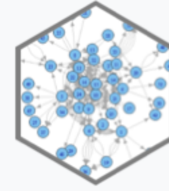
igraph
