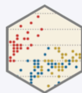
ggthemes
