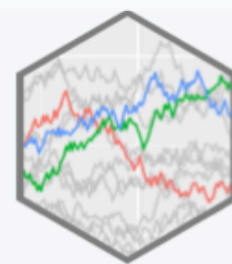
gghighlight
