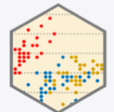
ggthemes
