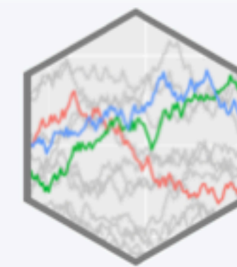
gghighlight
