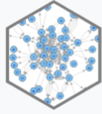
igraph
