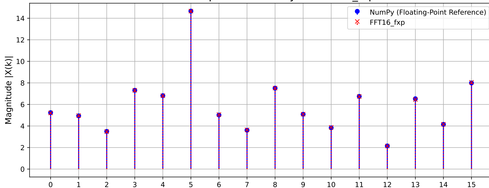
FFT16 Comparison: NumPy vs. FFT16_fxp
