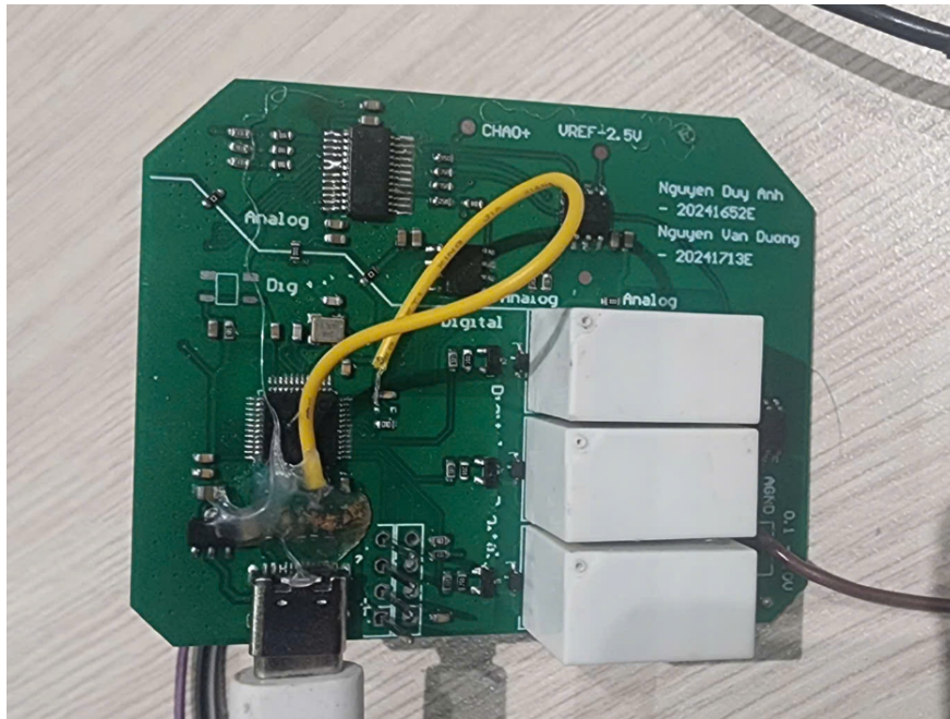
Hình 3.12: Bo mạch nguyên mẫu đã lắp ráp trong quá trình debug
