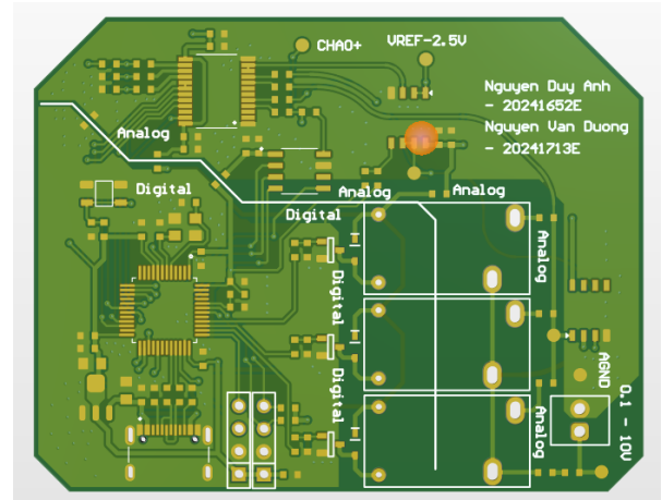
(b) Bề mặt PCB và footprint
