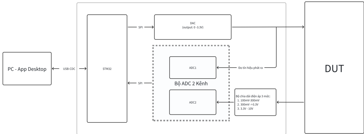
Hình 3.1: Kiến trúc tổng thể của hệ thống theo sơ đồ khối thiết kế
