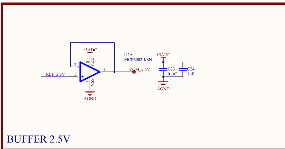
Hình 3.7: Sơ đồ nguyên lý buffer mức tham chiếu 2,5 V
