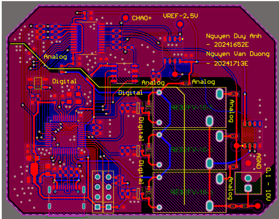
Hình 3.11: Layout các lớp đồng, via và vùng đổ đồng của PCB
