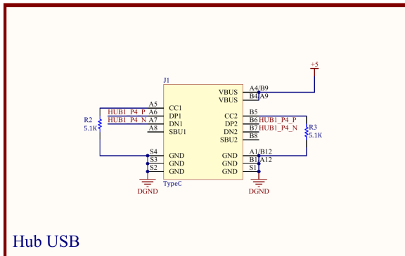
(a) Cổng USB Type-C và các đường D+/D-
