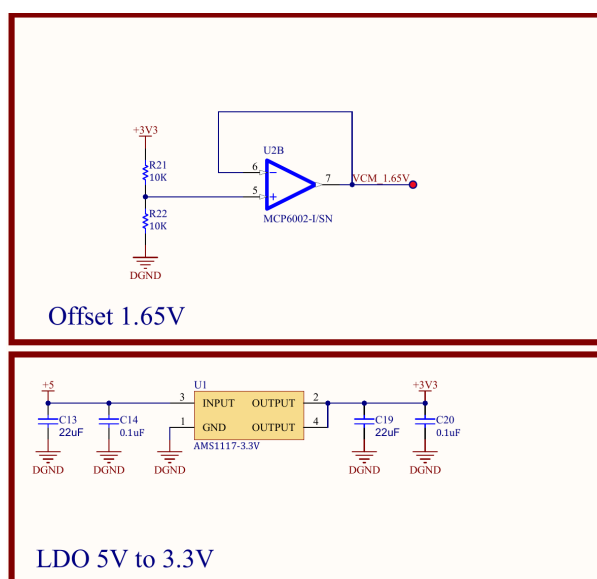
Hình 3.8: Sơ đồ nguyên lý offset 1,65 V và LDO 5 V xuống 3,3 V
