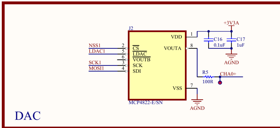
Hình 3.6: Sơ đồ nguyên lý DAC MCP4822 và giao tiếp SPI1
