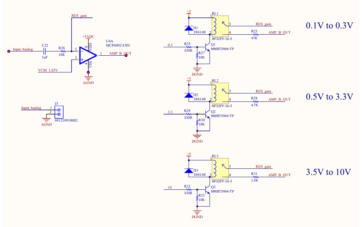
Hình 3.9: Sơ đồ nguyên lý AFE ghép AC, op-amp đảo và relay chọn ba dải đo CH2
