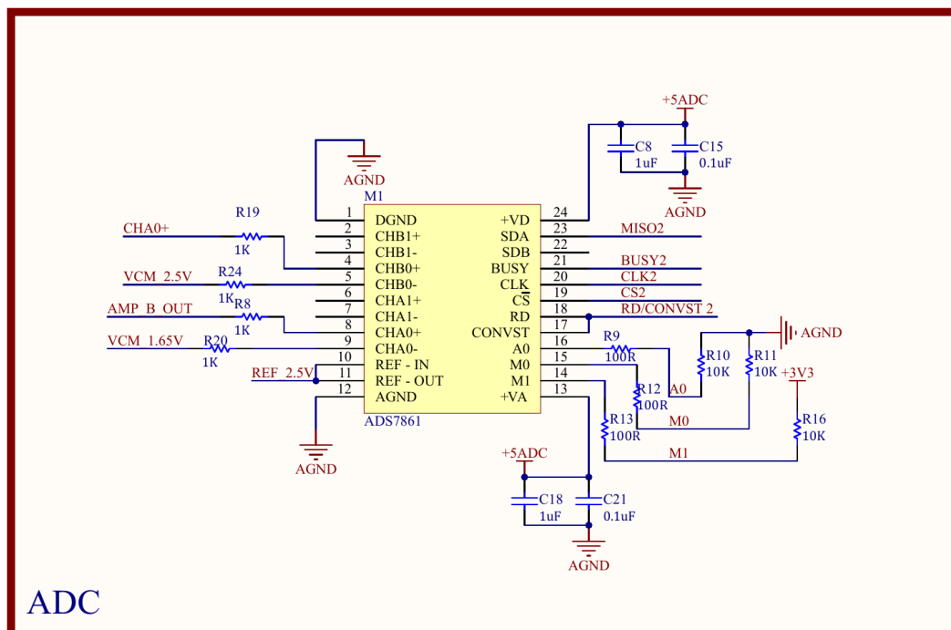
Hình 3.5: Sơ đồ nguyên lý ADS7861, nguồn analog, reference và các tín hiệu điều khiển
