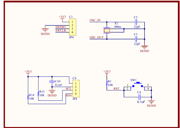
Hình 3.3: Sơ đồ nguyên lý khối giao tiếp, clock và debug
