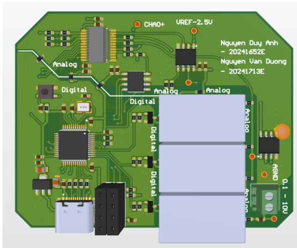
(a) Mô hình 3D có linh kiện
