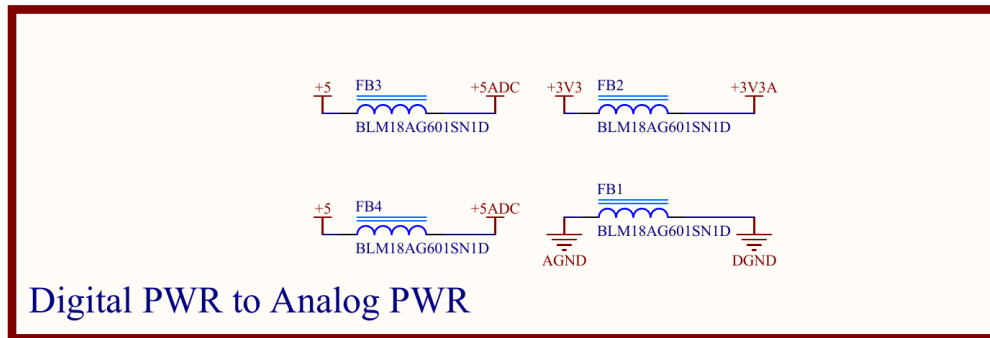
Hình 3.4: Ferrite bead phân tách nguồn số, nguồn ADC và miền mass analog–digital
