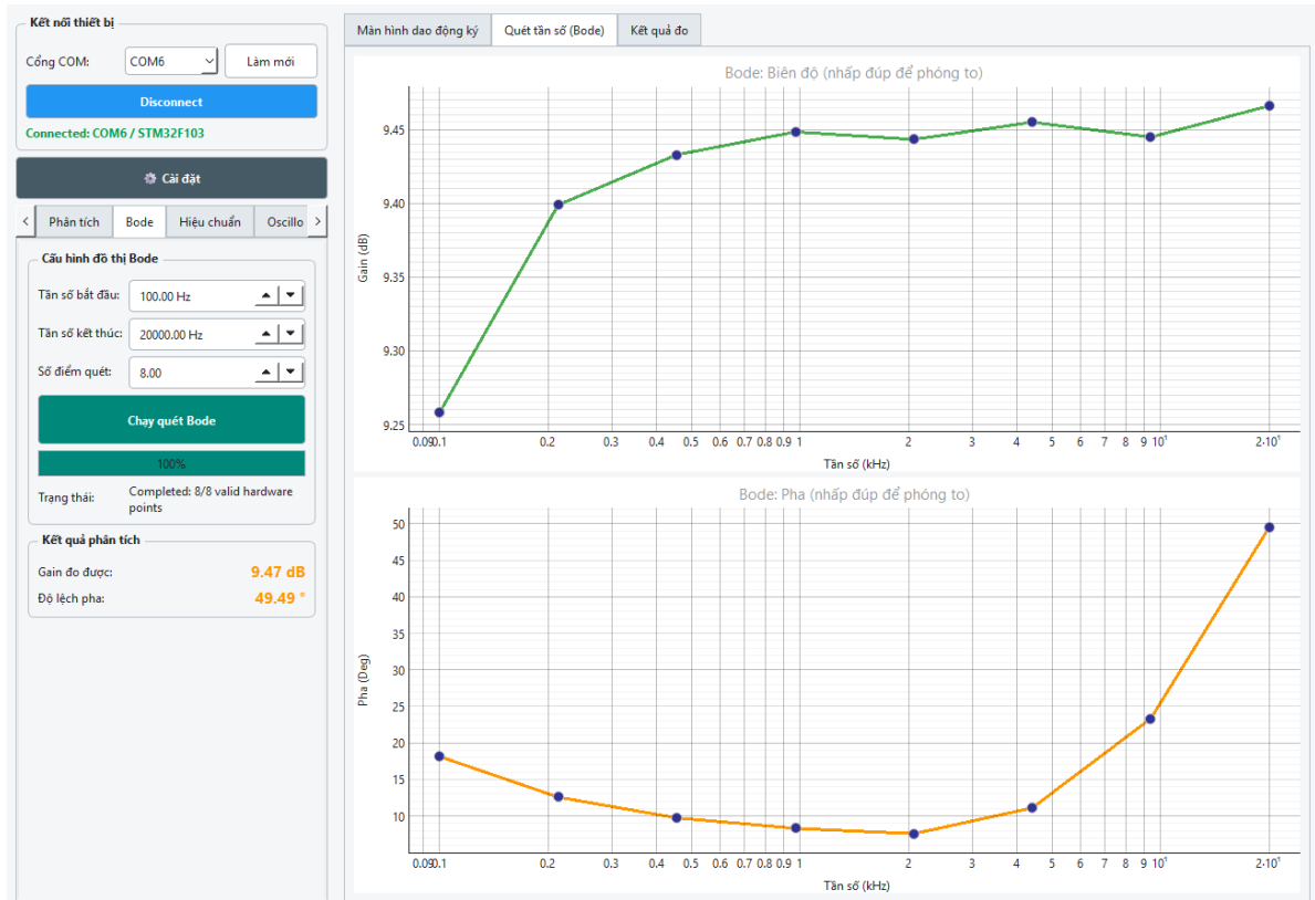
Hình 6.9: Đồ thị Bode đo trên phần cứng từ 100 Hz đến 20 kHz với DUT gain 3
