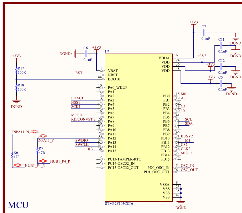
Hình 3.2: Sơ đồ nguyên lý khối STM32F103C8T6 và các tín hiệu ngoại vi chính
