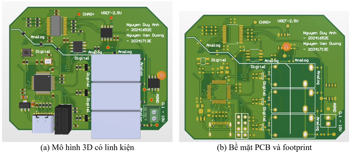
Hình 3.10: Mô hình bố trí PCB của thiết bị phân tích
