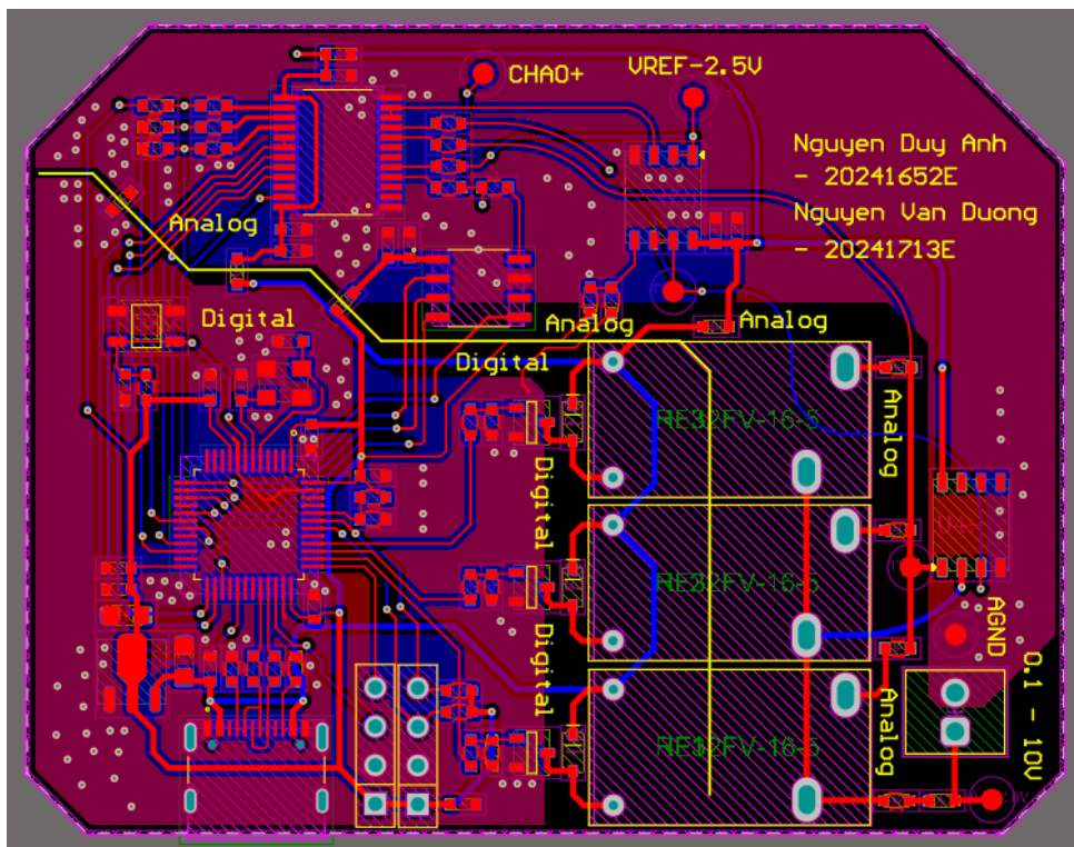
Hình 3.11: Layout các lớp đồng, via và vùng đồ đồng của PCB
