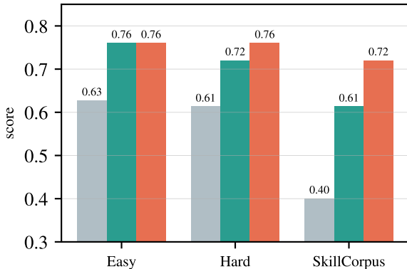
Hit@1
