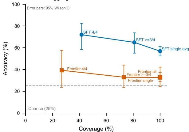
a Aggregation Frontier: SFT vs Frontier
