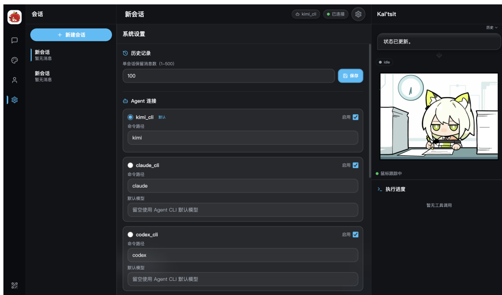
图 6: 系统设置页
