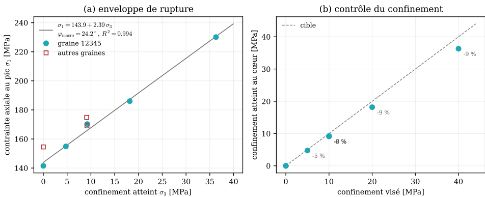
FIGURE 63 – Enveloppe du jeu de juillet. (a) Ajustement de Mohr-Coulomb des pics, angle macroscopique 24,2°. (b) Confinement atteint en fonction du confinement visé, inférieur de 5 à 9 %.
