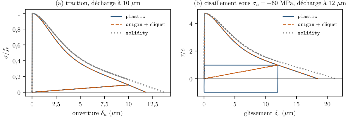
FIGURE 3 – Joint isolé, trois branches de décharge, rejoué. (a) Traction avec décharge à 10 μm. (b) Cisaillement sous \sigma_n = -60 MPa avec décharge à 12 μm : seule la branche plastic conserve un glissement résiduel.
