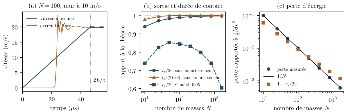
FIGURE 7 – Chaîne de N masses frappée à 10 m/s par le contact de Signorini, rejoué. La barre repart à 2v après 2L/c , et la seule perte, 1/N , est celle du premier toucher.
