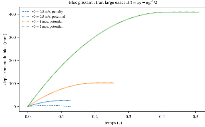
FIGURE 13 – Bloc glissant : déplacement contre en fonction du temps pour trois vitesses initiales, contact par potentiel et par pénalité nœud-face, solution exacte en trait large.
