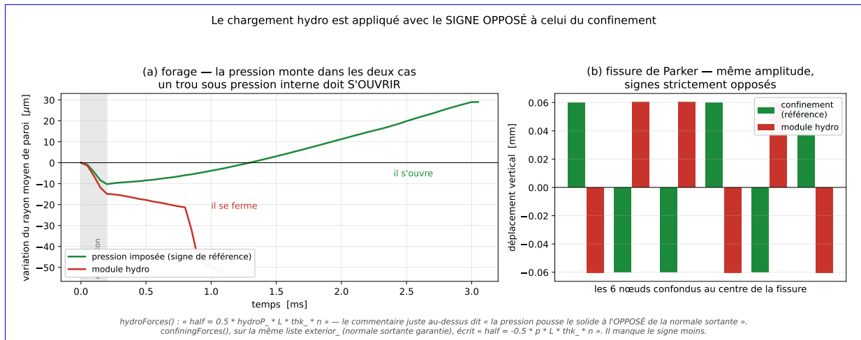
FIGURE 33 – Défaut de signe du 19 août 2026, figure d'archive. (a) La paroi rentre de 50 \mu\text{m} sous le module hydraulique et sort de 29 \mu\text{m} sous le confinement. (b) Déplacements des six nœuds centraux de la fissure de Parker : même amplitude, signes opposés.
