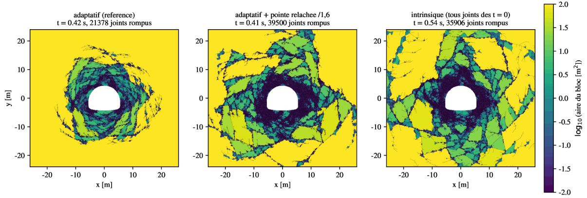
FIGURE 39 – Taille des blocs intacts (aire en échelle logarithmique) pour l’insertion adaptative, l’adaptative avec k_{tip} = 1,6 et l’intrinsèque : l’adaptative granule un anneau, les deux autres découpent des blocs polygonaux de quelques dizaines à quelques centaines de m^2 .
