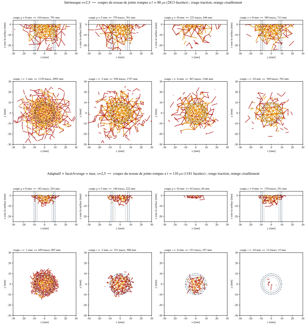
FIGURE 58 – Jumeau Kuru grossier de Kuru : traces des joints rompus, insertion intrinsèque à 80\ \mu\text{s} (haut) et adaptative avec critère du maximum à 110\ \mu\text{s} (bas).
