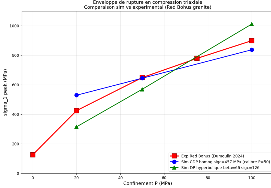
FIGURE 65 – Abaqus, lois continues : le modèle d’endommagement plastique calé à 50 MPa donne une enveloppe linéaire, le Drucker-Prager hyperbolique une courbure de sens contraire.
