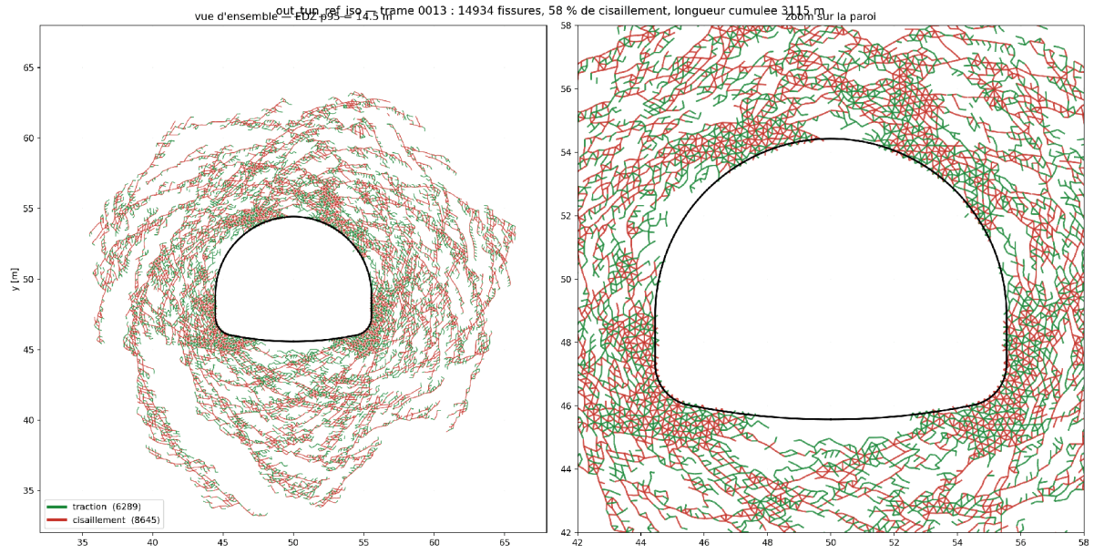
FIGURE 35 – Réseau de fissures du cas de référence, traction en vert et cisaillement en rouge : vue d'ensemble et zoom sur la paroi. L'anneau est classé en deux modes, selon la part dominante (traction en vert, 6 289 ; cisaillement en rouge, 8 645), et non en trois comme le texte. Anneau quasi circulaire et granulé à l'échelle de l'élément près de la paroi.
