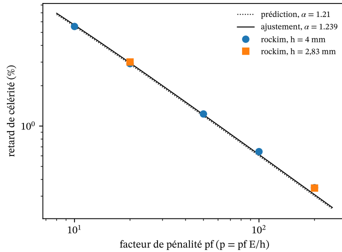
FIGURE 14 – Retard de célérité de l'onde contre le en fonction du facteur de pénalité intrinsèque, sur deux maillages, avec la prédiction écrite avant le balayage et l'ajustement.
