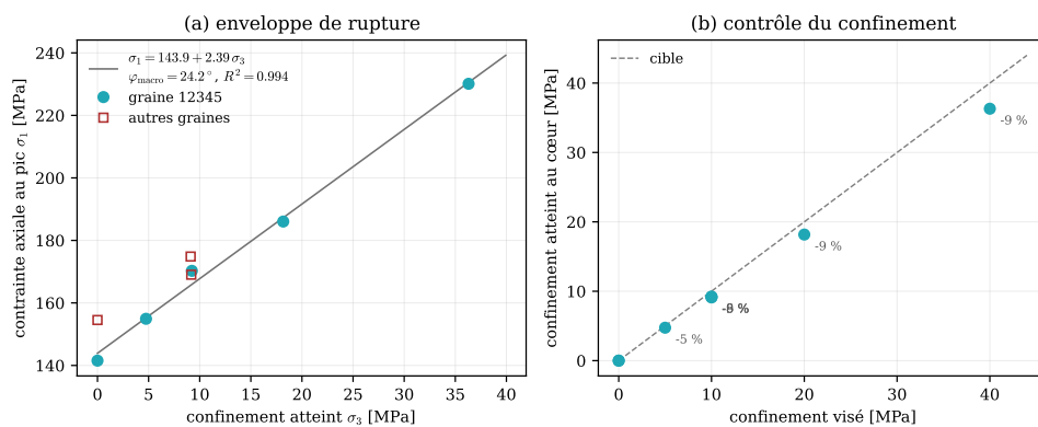
FIGURE 63 – Enveloppe du jeu de juillet. (a) Ajustement de Mohr-Coulomb des pics, angle macroscopique 24,2^\circ . (b) Confinement atteint contre en fonction du confinement visé, sous-tiré inférieur de 5 à 9 %.
