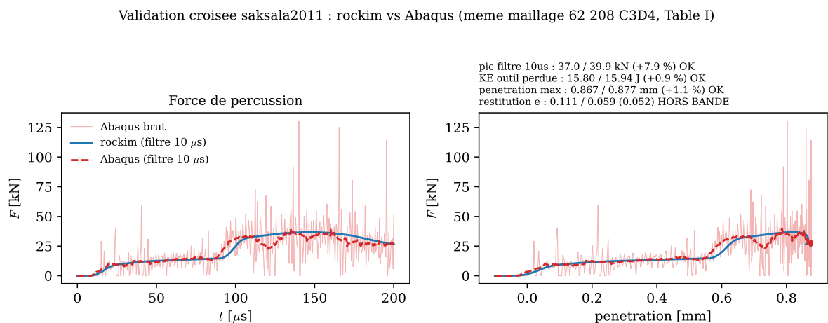
FIGURE 61 – Validation croisée Comparaison de code à code entre rockim et Abaqus/Explicit, loi de Saksala 2011, même maillage : force de percussion filtrée contre le en fonction du temps et de la pénétration.
