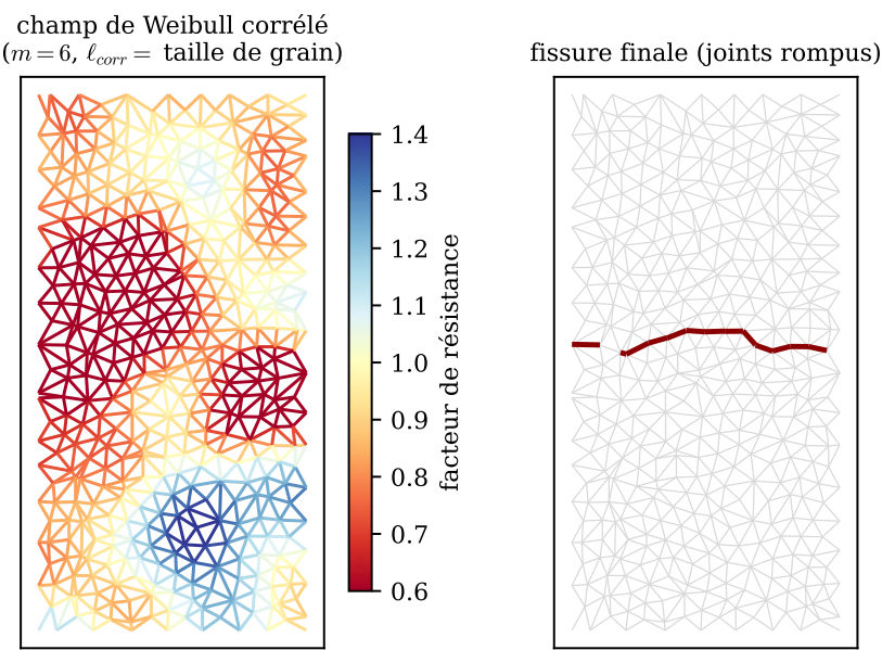
FIGURE 66 – Champ de Weibull corrélé sur les joints ( m = 6 , longueur de corrélation égale à la taille de grain) et fissure de traction finale, qui suit la bande la plus faible.
