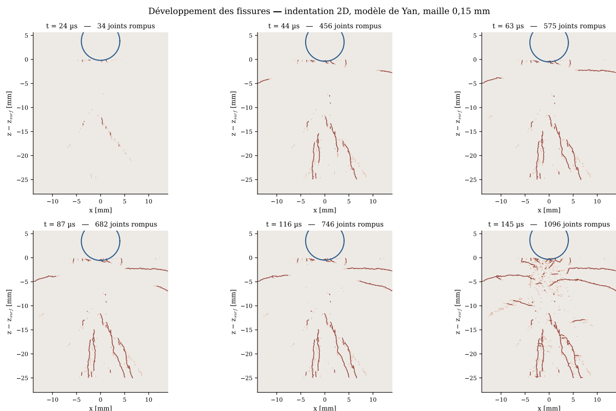
FIGURE 60 – Indentation 2D d'un bouton sphérique, modèle de Yan, maille de 0,15 mm : fissures médianes, puis latérales, puis broyage sous le bouton à la décharge.
