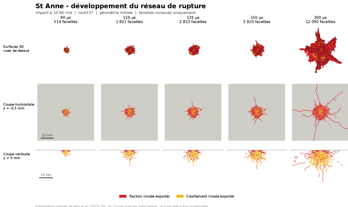
FIGURE 50 – Réplique St Anne : développement du réseau de facettes rompues de 90 à 300 \mu s, vu de dessus, en coupe horizontale à -0,5 mm et en coupe verticale ; couleur selon le mode de rupture.
