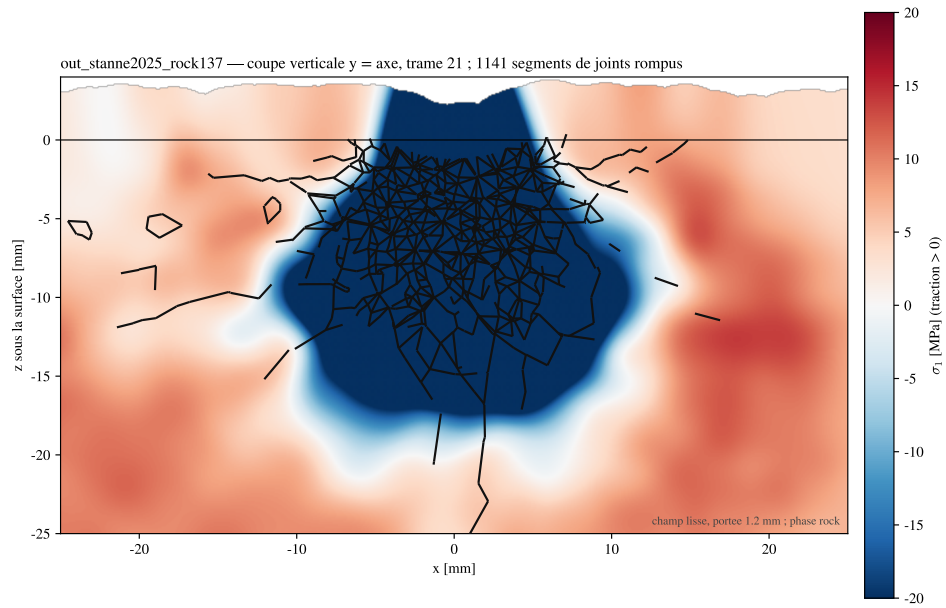
FIGURE 54 – Contrainte principale majeure (traction positive) en coupe verticale par l'axe à 300 \mu\text{s} , avec les traces des joints rompus : noyau comprimé sous l'insert, couronne en traction.
