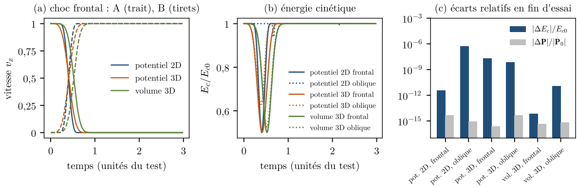
FIGURE 6 – Collision de deux corps par le contact, rejoué. (a) Vitesses au choc frontal. (b) Énergie cinétique. (c) Écarts relatifs finaux d'énergie cinétique et de quantité de mouvement.
