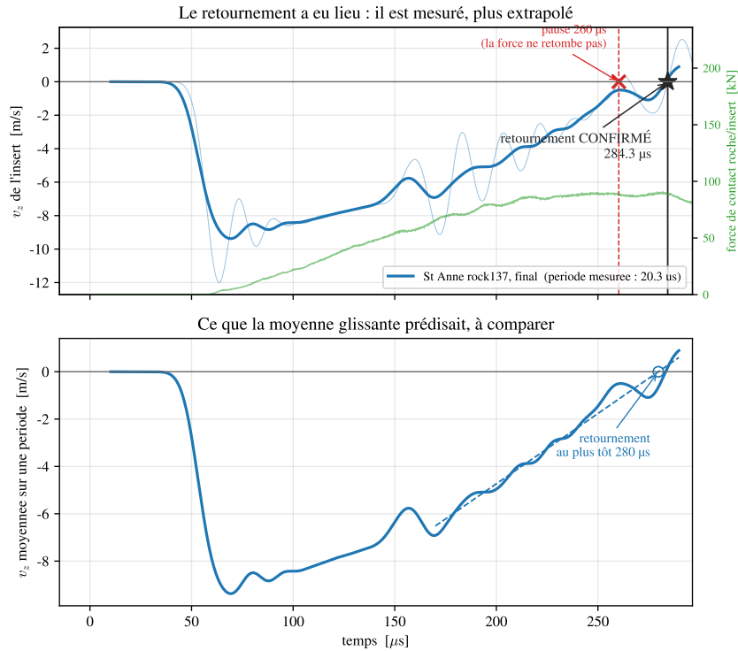
FIGURE 56 – Datation de la fin de charge : la vitesse de l'insert s'annule à 260 \mu\text{s} sans décharge, puis s'inverse à 284,3 \mu\text{s} .
