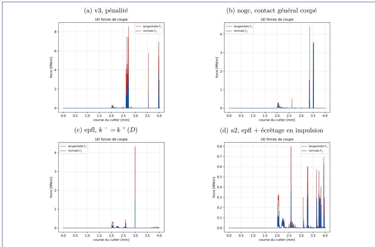
FIGURE 45 – Forces de coupe tangentielle (rouge) et normale (bleu) en fonction de la course, calculs d'août 2026, planches d'archive recadrées : (a) v3 ; (b) contact général coupé ; (c) pénalité de compression de Ghesquière-Diérickx et al. ; (d) même pénalité et écrêtage en impulsion.
