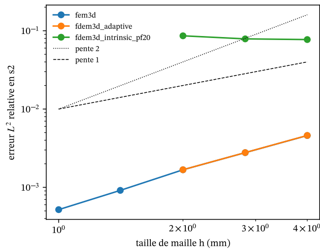
FIGURE 12 – Onde dans une barre : erreur L^2 du déplacement à mi-longueur contre en fonction de la taille d'élément, pour les éléments finis et les deux schémas d'insertion.
