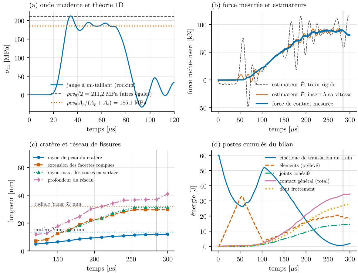
FIGURE 49 – Réplique St Anne : (a) onde à la jauge et théorie unidimensionnelle ; (b) force insert-roche mesurée et estimateurs ; (c) croissance du cratère et du réseau ; (d) postes du bilan d'énergie. Trait vertical : fin de charge.
