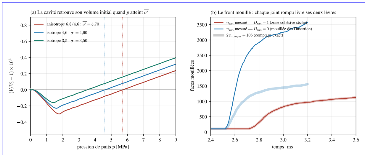
FIGURE 27 – Contrôles du couplage. (a) Volume relatif de la cavité en fonction de la pression : il revient à sa valeur initiale quand la pression égale la contrainte moyenne in situ. (b) Front mouillé : deux lèvres par joint rompu à D_{wet} = 1 .
