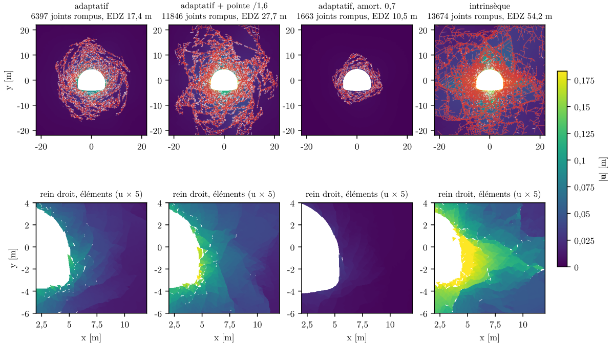
FIGURE 43 – Rejeu sur maillage réduit (binaire f0209ef0209ef ), quatre variantes à 0,23 s après le début du relâchement. En haut, norme du déplacement sur la configuration déformée et joints rompus (rouge : cisaillement ; blanc : traction). En bas, rein droit en rendu éléments, déplacements amplifiés 5 fois.
