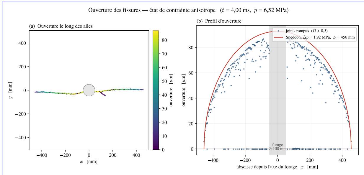
FIGURE 28 — Ouverture des fissures à t = 4 ms, état anisotrope, reconstruite lèvres à lèvres, et ellipse de Sneddon ( \Delta p = 1,92 MPa, L = 456 mm) : 89,0 \mu\text{m} mesurés pour 92,8 \mu\text{m} prédits. Les points à ouverture nulle sont des joints refermés.
