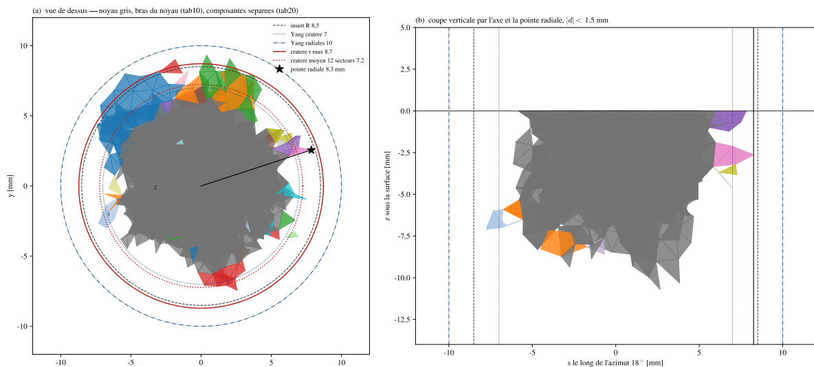
FIGURE 57 – Réplique Kuru, maillage fin, à 180 \mu\text{s} : réseau connecté vu de dessus et en coupe ; noyau dense de 7 à 9 mm, pas d'étoile radiale.
