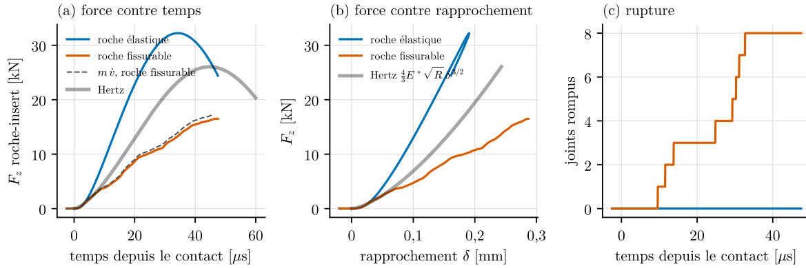
FIGURE 59 – Impact d’un insert en carbure sur roche élastique et fissurable, 50 \mu s , rejoué : force de contact contre comparée à la solution de Hertz ; le contact maillé est trop raide ; en roche fissurable , l’adoucissement des joints l’assouplit amortie , la force baisse avant toute rupture.
