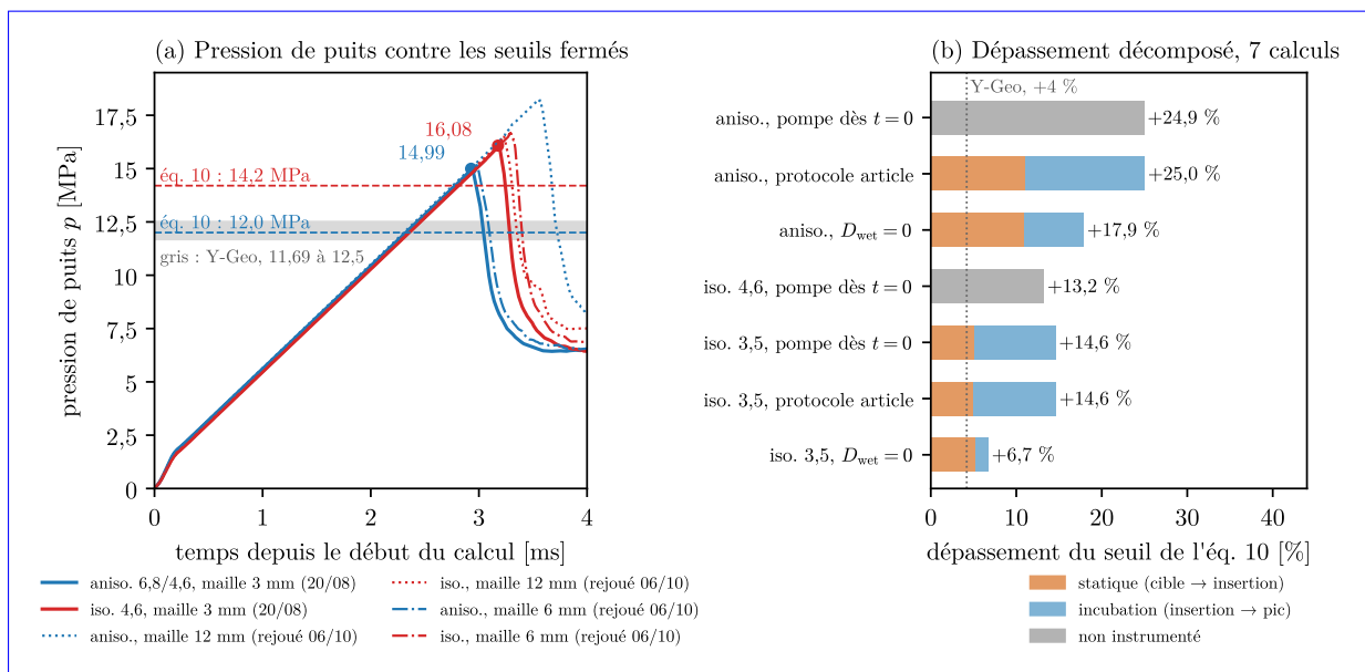
FIGURE 29 — (a) Pression de puits, calculs d'août à 3 mm (traits épais), rejeux du 6 octobre à 12 mm (pointillés) et 6 mm (tirets-points) ; Hubbert et Willis en tirets, Y-Geo en gris. (b) Dépassement du seuil des sept calculs d'août, statique et incubation.
