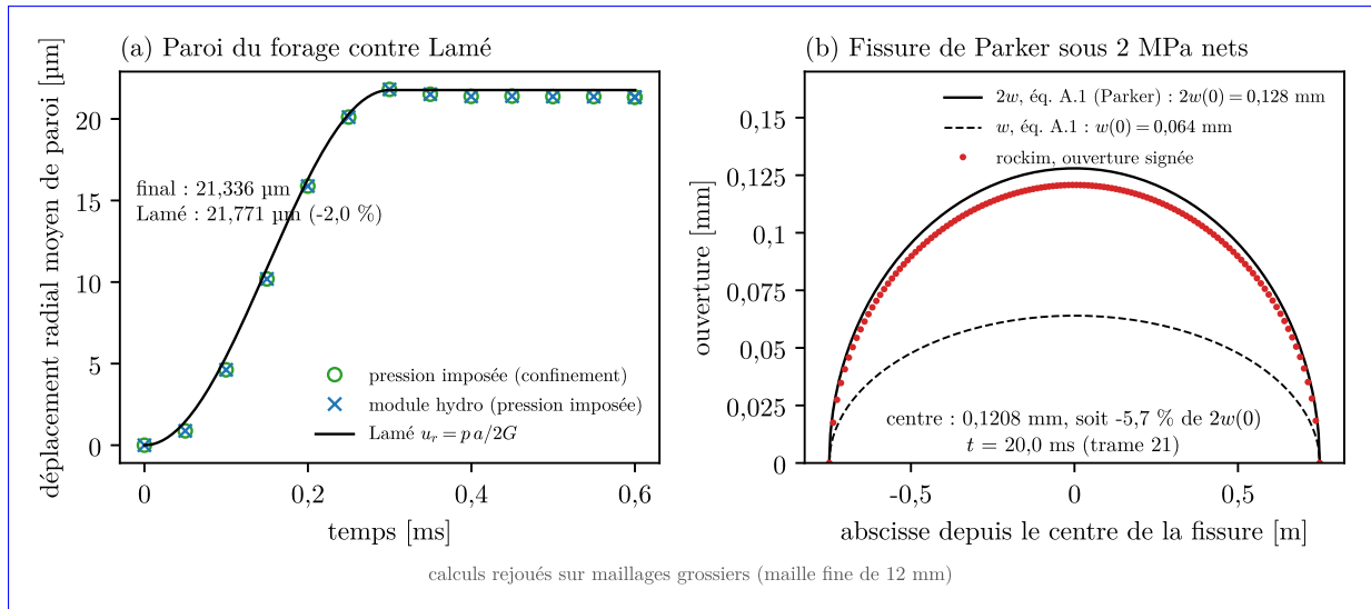
FIGURE 26 – Vérifications rejouées le 6 octobre 2026 (binaire f0209ef). (a) Paroi d'un forage sous 12 MPa : les deux chemins de chargement se superposent, à -2,0 % de Lamé. (b) Fissure de Parker sous 2 MPa nets : ouverture à -5,65 % de 2w au centre.
