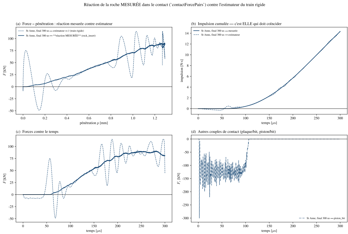
FIGURE 55 – Réplique St Anne : force de contact insert-roche mesurée contre l'estimateur du train rigide, en fonction de la pénétration et du temps, impulsions cumulées et autres paires de contact.
