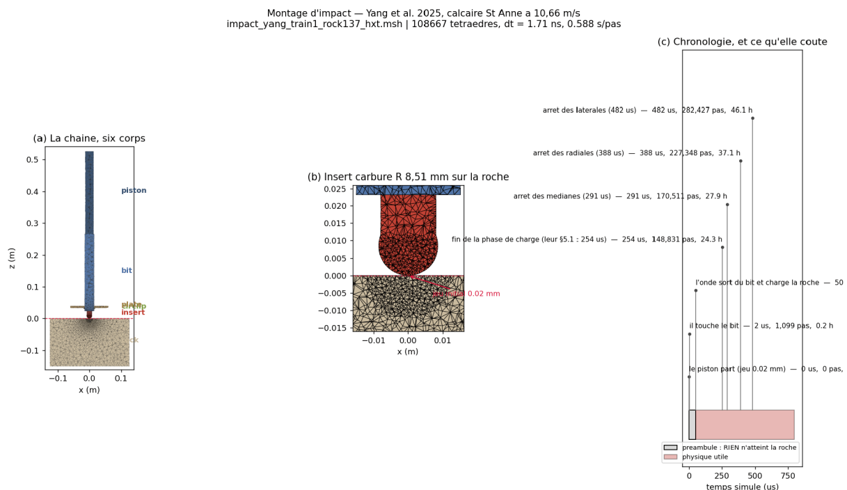
FIGURE 48 – Montage de la réplique St Anne : chaîne de six corps, insert en carbure posé à 0,02 mm de la roche, et coût en temps de calcul des événements de la chronologie.
