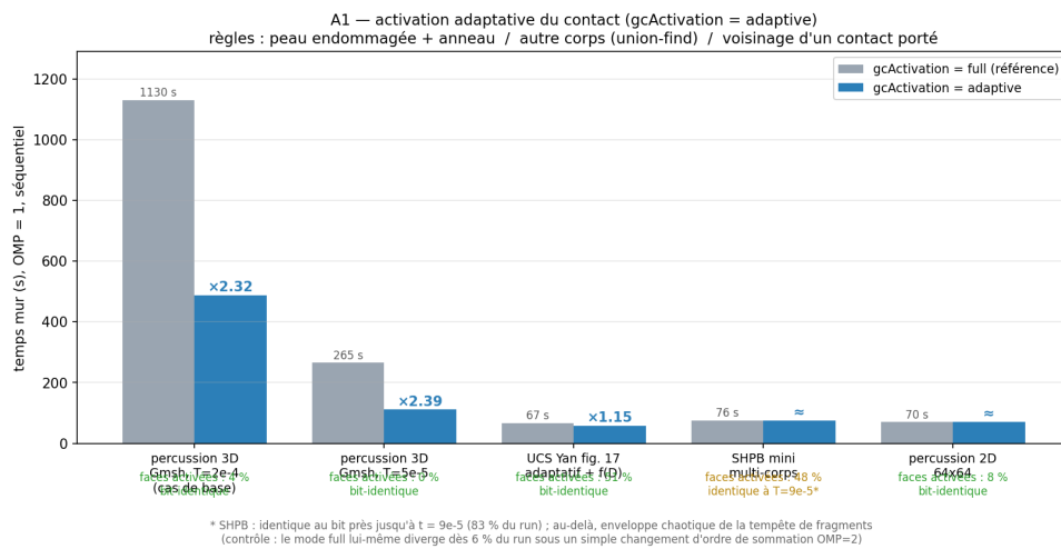
FIGURE 67 – Temps de calcul avec et sans activation adaptative du contact sur cinq cas, à un fil, avec la part de faces activées.
