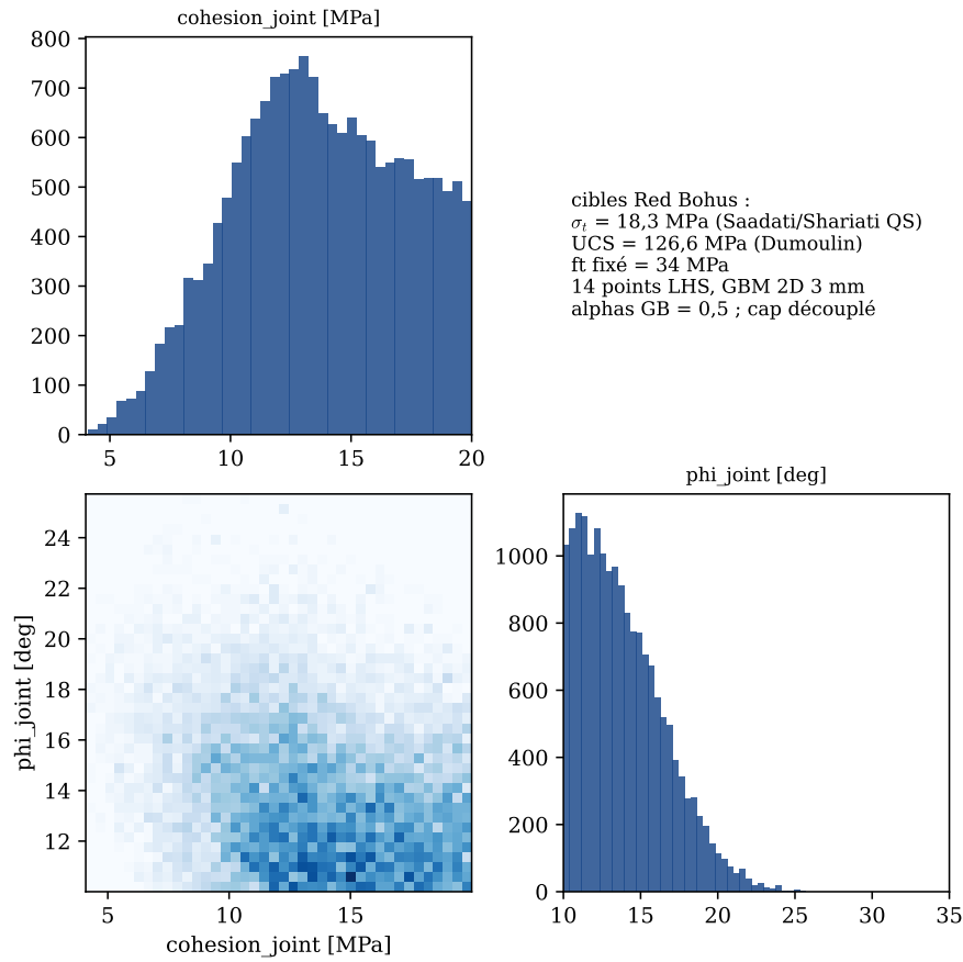
FIGURE 62 – Postérieur Loi a posteriori de la calibration de juillet, modèle à grains 2D : angle de frottement des joints médian 13,4^\circ , tronqué par la borne a priori ; cohésion peu contrainte.
