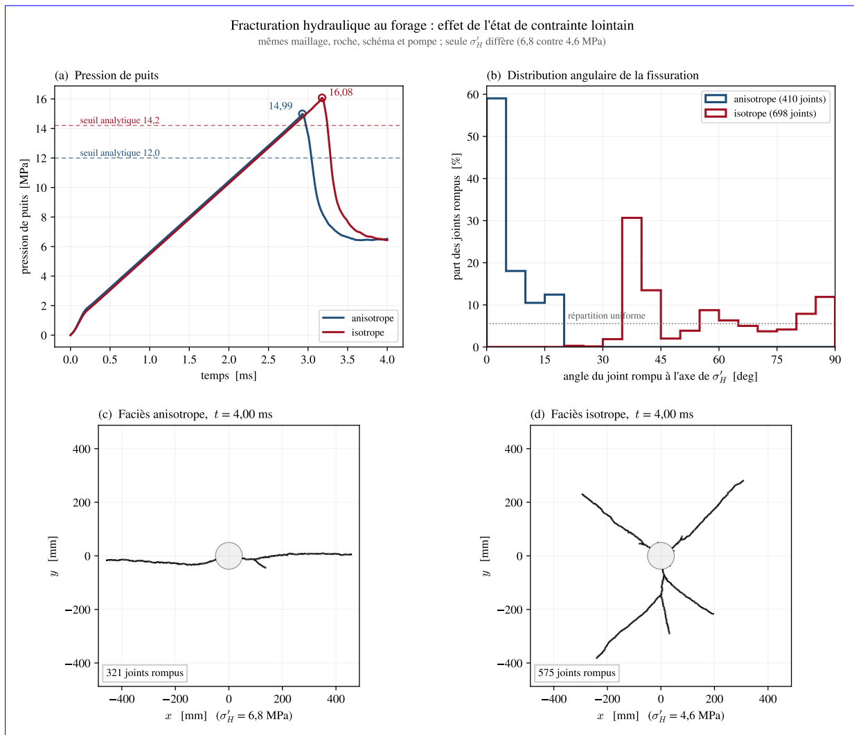
FIGURE 31 – Effet de l'état de contrainte lointain : (a) pression de puits et seuils analytiques de 12,0 et 14,2 MPa ; (b) distribution angulaire des joints rompus ; (c, d) à 4 ms, deux ailes en anisotrope (321 joints rompus), étoile radiale en isotrope (575).
