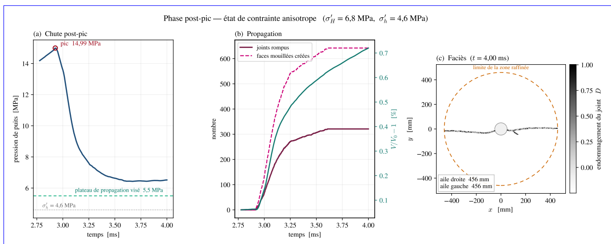
FIGURE 32 – Phase post-pic, état anisotrope : (a) la pression s'infléchit vers 6,5 MPa, au-dessus du plateau de 5,5 MPa de l'article ; (b) joints rompus, faces mouillées et volume de la cavité ; (c) faciès, les ailes atteignant la limite de la zone raffinée.
