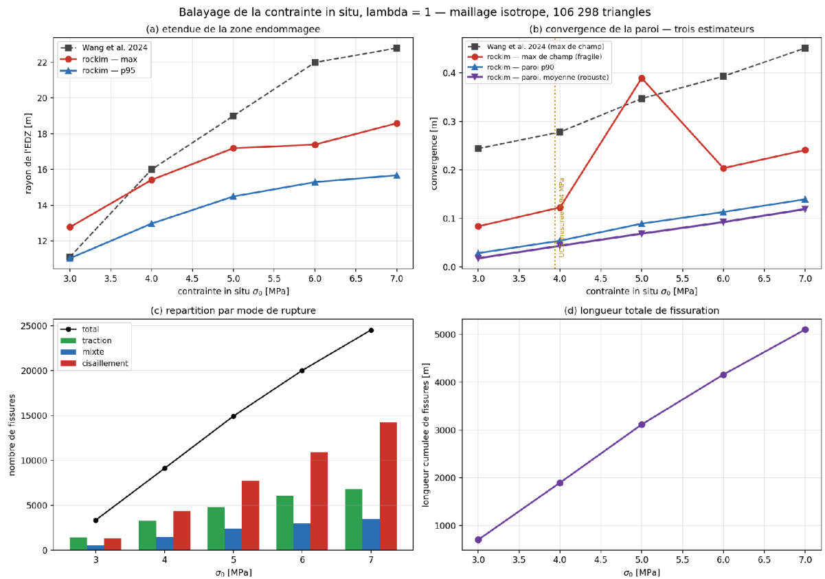
FIGURE 36 – Balayage de la contrainte in situ ( \lambda = 1 ) : (a) rayon d'EDZ comparé aux , maximum et quantile 95 %, et valeurs lues chez Wang et al. , ; (b) convergence : maximum du champ, quantile à 90 % et moyenne de paroi selon trois estimateurs, répartition des ; (c) modes et ; (d) longueur fissurée.
