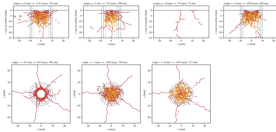
FIGURE 52 – Réplique St Anne à 300 \mu s : traces exactes des facettes rompues dans sept plans de coupe ; rouge traction, orange cisaillement.
