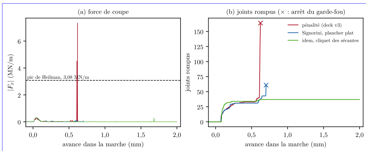
FIGURE 46 – Rejeu du deck v3 : (a) force de coupe |F_x| et pic de Heilman ; (b) joints rompus, en fonction de l'avance de l'arête au-delà de la face d'entaille. Les croix marquent l'arrêt par le garde-fou d'énergie.
