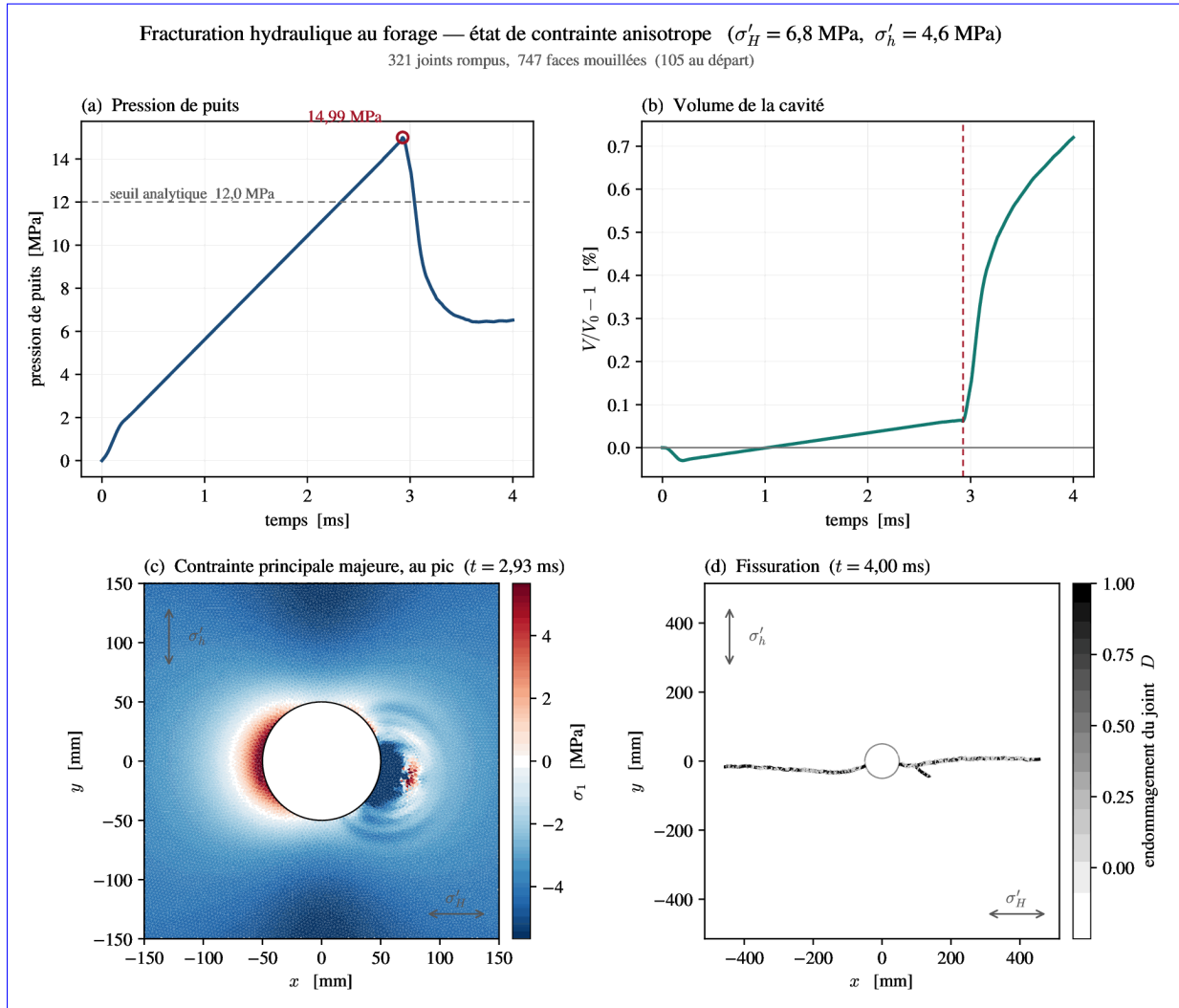
FIGURE 30 – Forage sous injection, état anisotrope : (a) pression de puits, pic de 14,99 MPa contre 12,0 MPa (Hubbert et Willis) ; (b) volume de la cavité ; (c) contrainte principale majeure au pic ; (d) fissuration à 4 ms, deux ailes de 456 mm sur l'axe de \sigma'_H .
