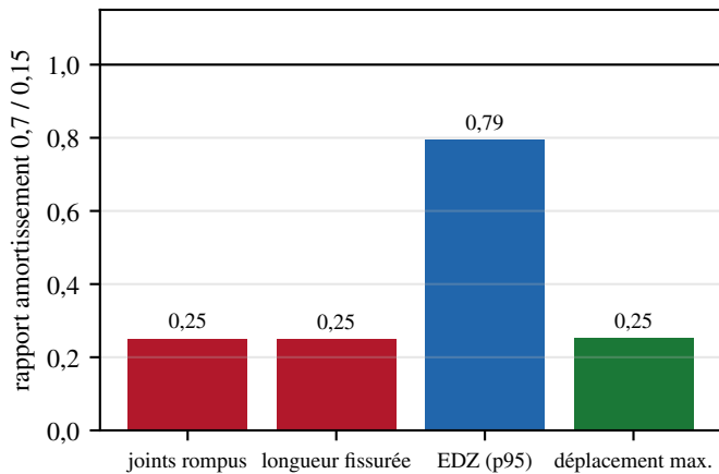
(d) effet de dampingLocal (maillage de fumée)
