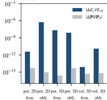
(c) écarts relatifs en fin d'essai
