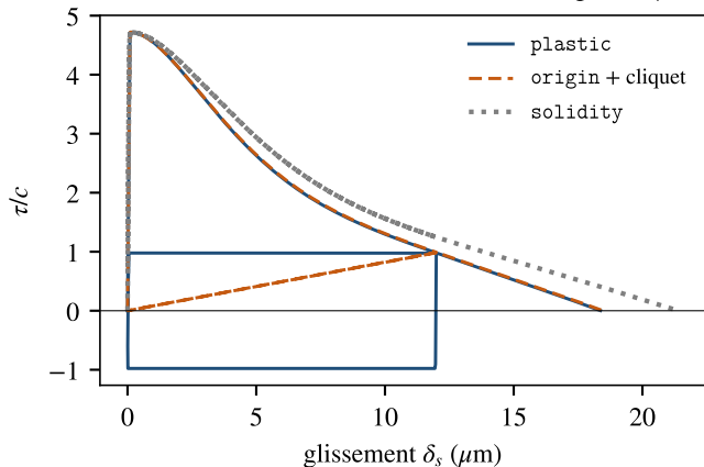
(b) cisaillement sous \sigma_n = -60 MPa, décharge à 12 \mu\text{m}
