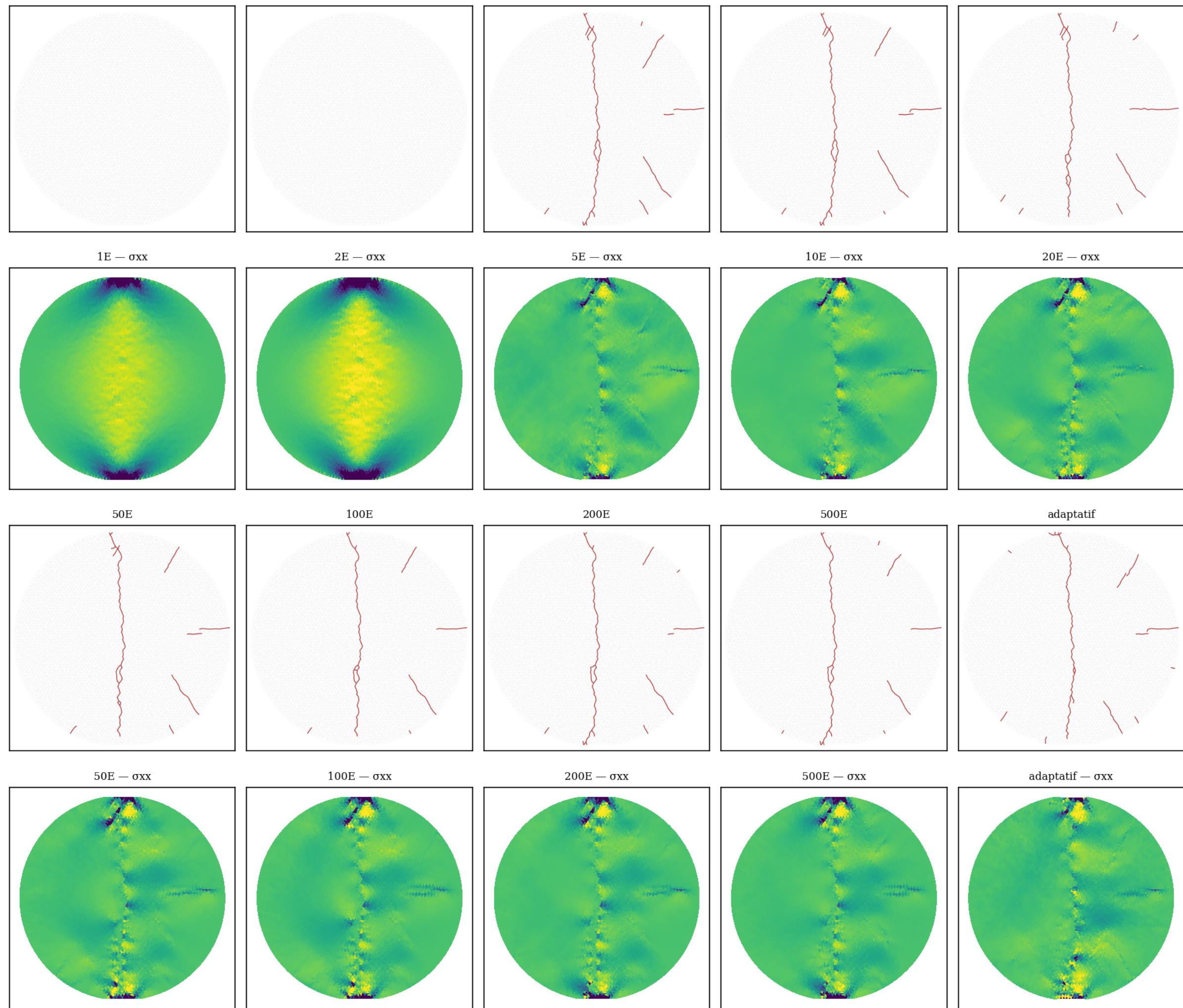
Fig. 12 — faciès et champs \sigma_{xx} post-pic, 1E-500E + adaptatif
