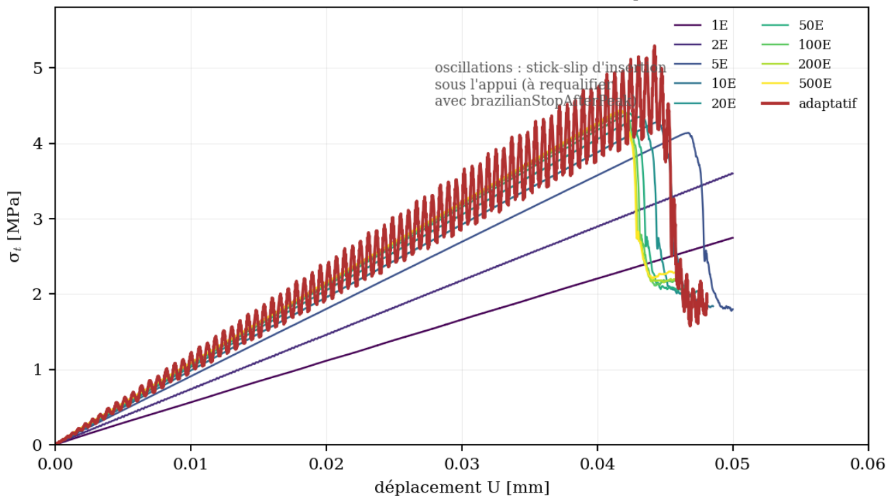
(a) brésilien, loi f(D) — famille 1E-500E vs adaptatif
