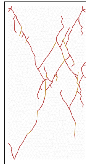
Faciès UCS (haut, fig. 18) et triaxiaux adaptatifs (bas, fig. 20) — rouge intra-grain, ocre joints
